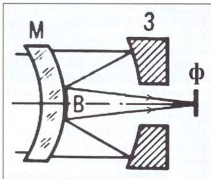
(6) Оптическая схема менискового телескопа. З – главное зеркало телескопа; М – мениск с двумя сферическими поверхностями; В – вторичное зеркало, направляющее и фокусирующее пучок света от небесного объекта на фотокатод приёмника света
