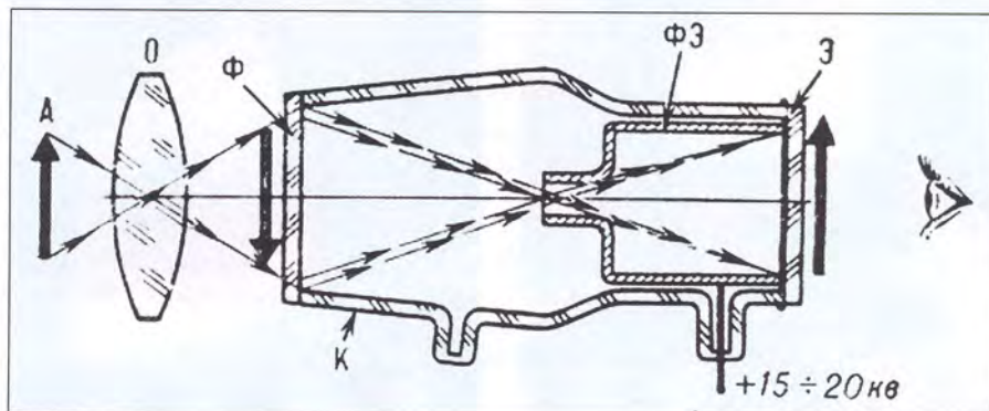
(3) Схема работы однокамерного ЭОПа
