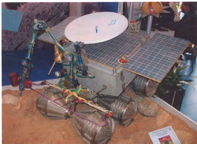
Действующая модель планетохода второго поколения, разработанная специалистами НПО им. С. Лавочкина
