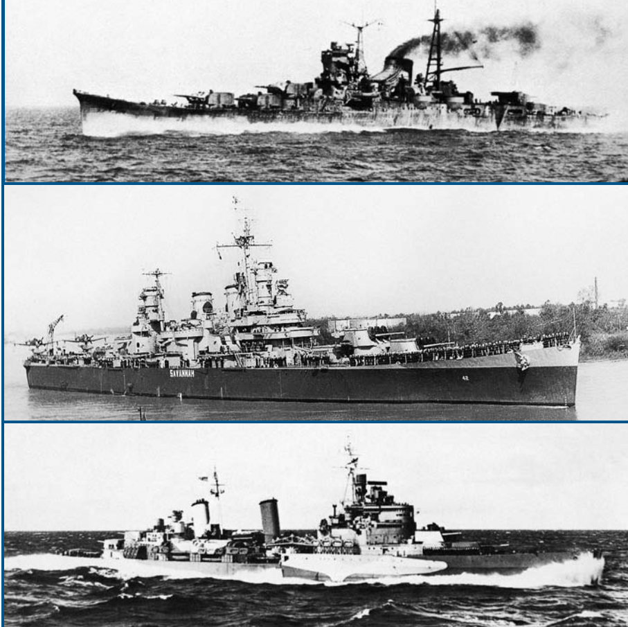
Три попытки построить самый мощный «лондонский» лёгкий крейсер (сверху вниз): японский «Могами», американский «Саванна» типа «Бруклин», британский «Белфаст»
