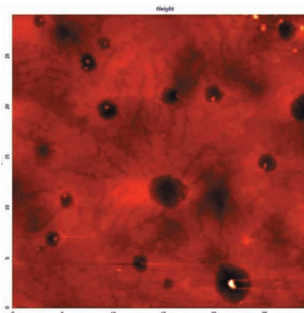
Микрофотография поливинилспиртовой плёнки, содержащей иммобилизованный фермент. Агрегаты фермента, взаимодействующие с компонентами полимерной композиции, становятся центрами структурообразования
