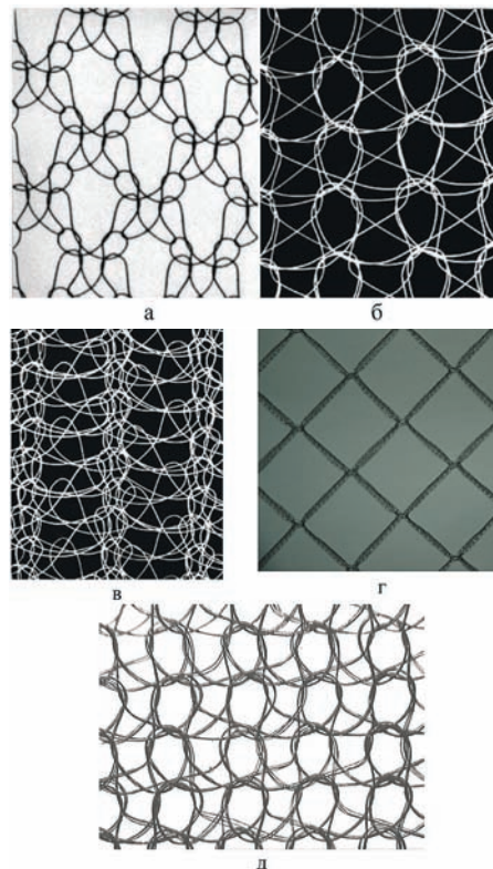
Микрофотографии различных металлических сетеполотен:
