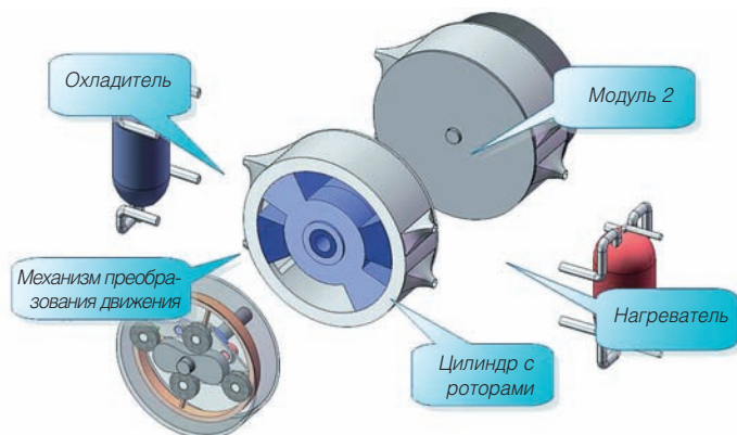
Конструкция роторно-лопастного двигателя с внешним подводом теплоты
