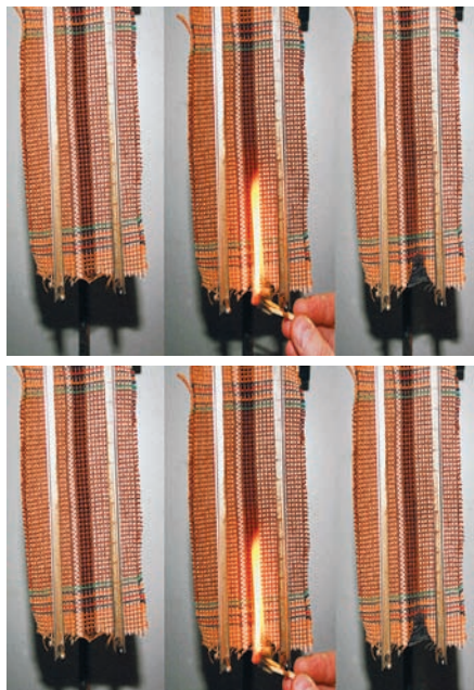
Оценка горючести текстильного материала. Исходная ткань (внизу) — после поджигания сгорает практически полностью. Ткань, содержащая огнезамедлительную систему (вверху), при удалении источника огня — затухает
