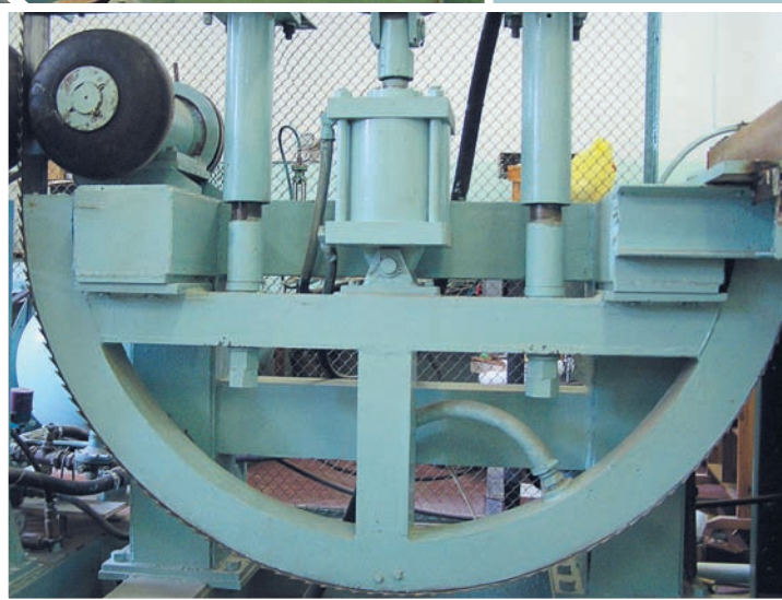
Рис. 4. Ленточнопильный станок, общий вид и агрегаты
