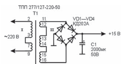
Рис. 4. Электрическая схема мощного источника питания
