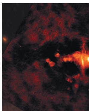
Радиотелескоп VLA в Мексике в длинных радиоволнах
