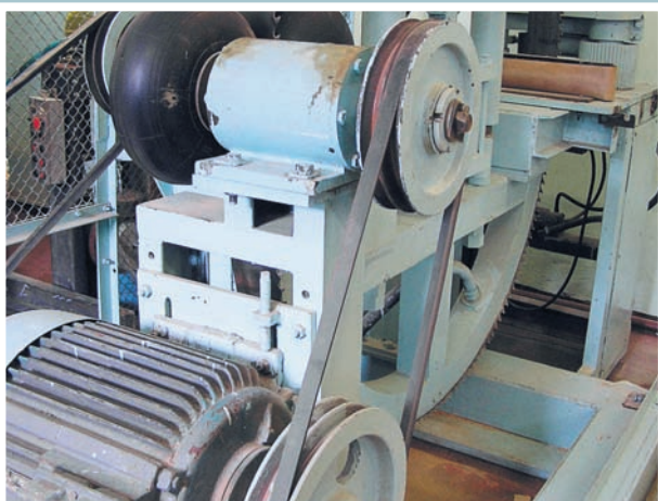
Электродвигатели и ременные передачи привода пилы
