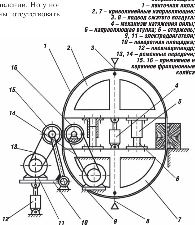
Рис. 2. Принципиальная схема узла резания ленточнопильного станка с пилой, движущейся по криволинейным аэростатическим направляющим:
