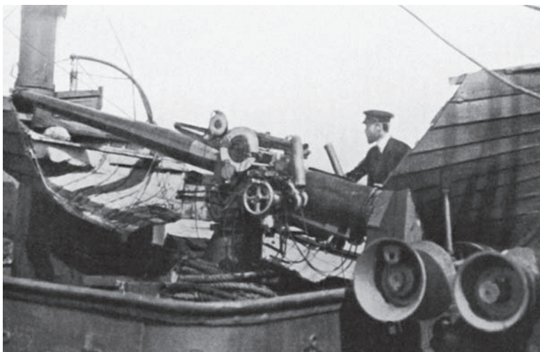
Замаскированная под шлюпку 12-фунтовая пушка «Пенхёрста» в обычном (слева) и боевом (справа) положениях
