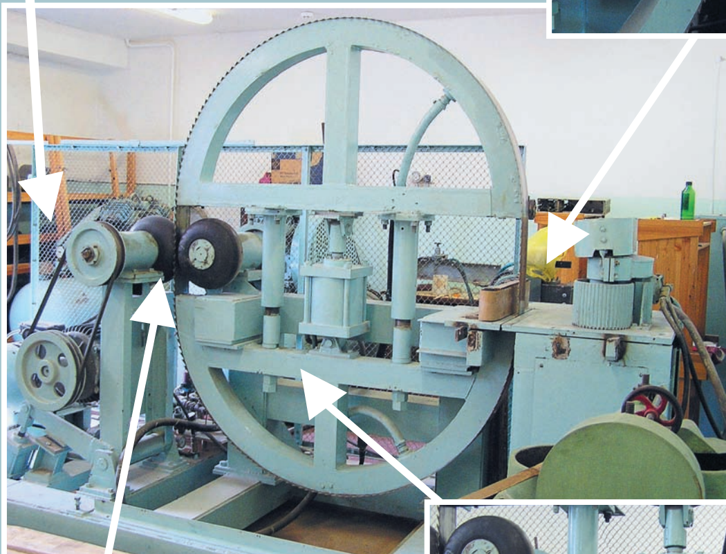
Приводные фрикционные колёса
