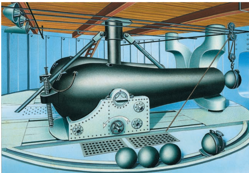
Броненосный корабль северян «Монитор», 1862 г.: водоизмещение — 987 т. Скорость — 7 узлов, вооружение: 2 — 280-мм, мощность силовой установки — 640 л.с., бронирование: пояс — 400 мм, башня — 200 мм, палуба — 25 мм, длина — 52,5 м, ширина — 12,5 м, осадка — 3 м
