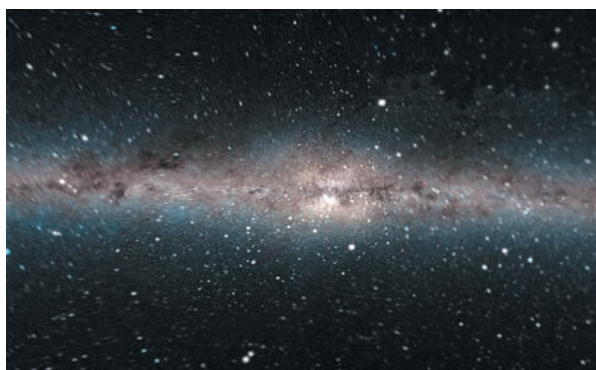
Настройка на инфракрасный диапазон существенно просветляет взгляд астронома
