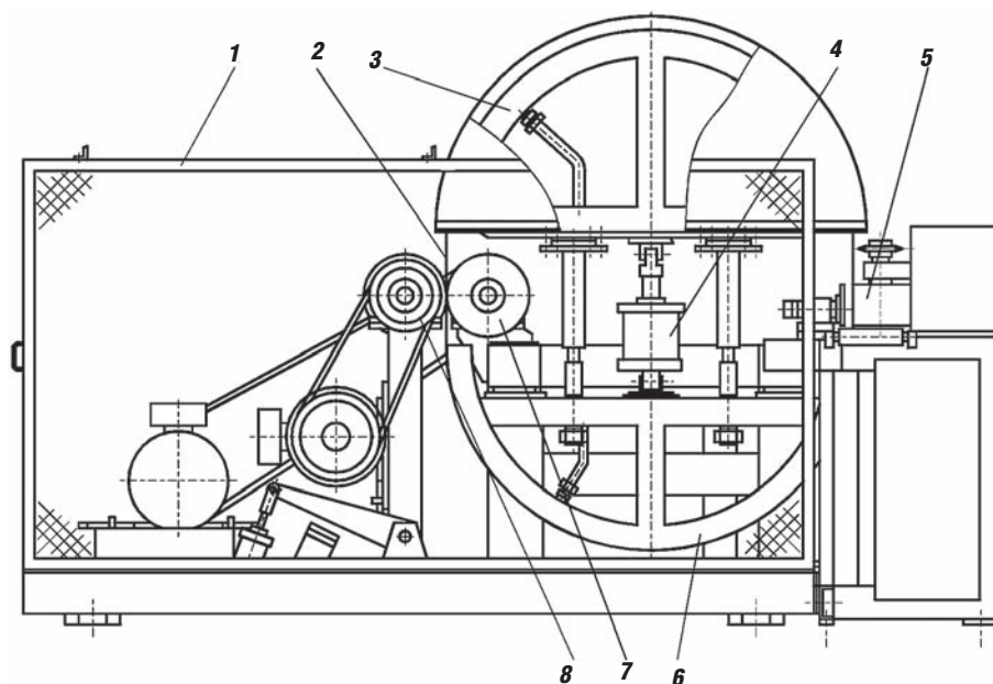
Рис. 3. Конструкция ленточнопильного станка с пилой, движущейся по криволинейным аэростатическим направляющим: 1 – ограждение; 2 – пила; 3, 4 – верхняя и нижняя криволинейные аэростатические направляющие; 5 – механизм натяжения пилы; 6 – механизм подачи распиливаемого материала; 7, 8 – приводные фрикционные колёса
