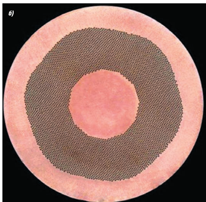
Рис. 3. Поперечные сечения низкотемпературных сверхпроводников: а) на базе интерметаллического соединения Nb_3Sn ; б) на основе сплава NbTi
