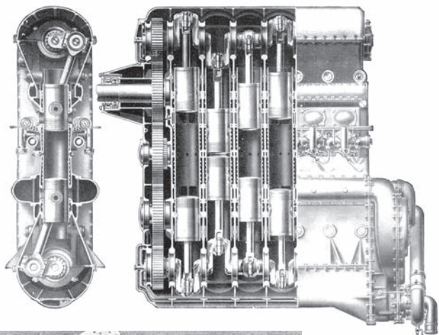
Двухтактный авиационный дизель JUMO «двухсотой» серии
