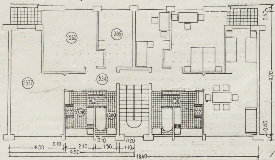
94. Типовой проект трехкомнатной квартиры. Стройком РСФСР
