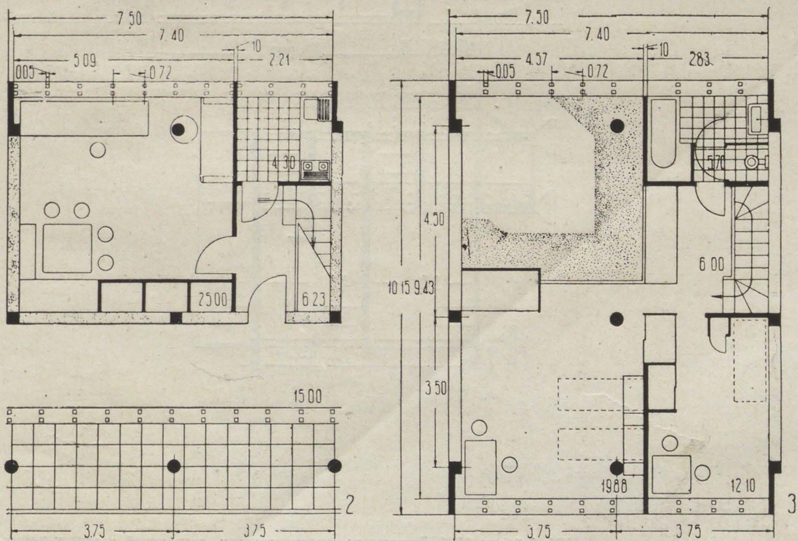
130. 2-й дом СНК. Планы квартиры—тип H. 2-й 3-й этажи. М. Я. Гинзбург и И. Ф. Милинис
