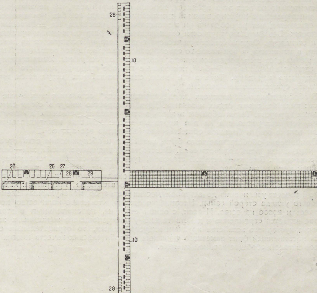
189 и 190. Дом-коммуна. Планы 5-го и 6-го этажей. Стройком РСФСР. М. О. Барщ и В. Н. Владимиров
