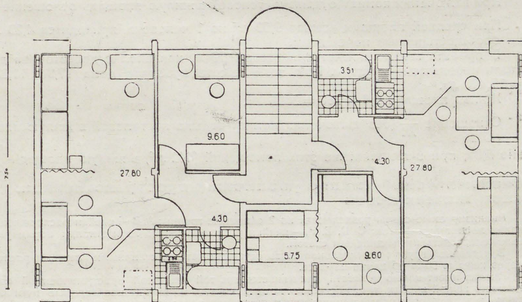
96. Типовой проект двухкомнатной квартиры — тип В. Планы 1-го и 2-го этажей. Стройком РСФСР
