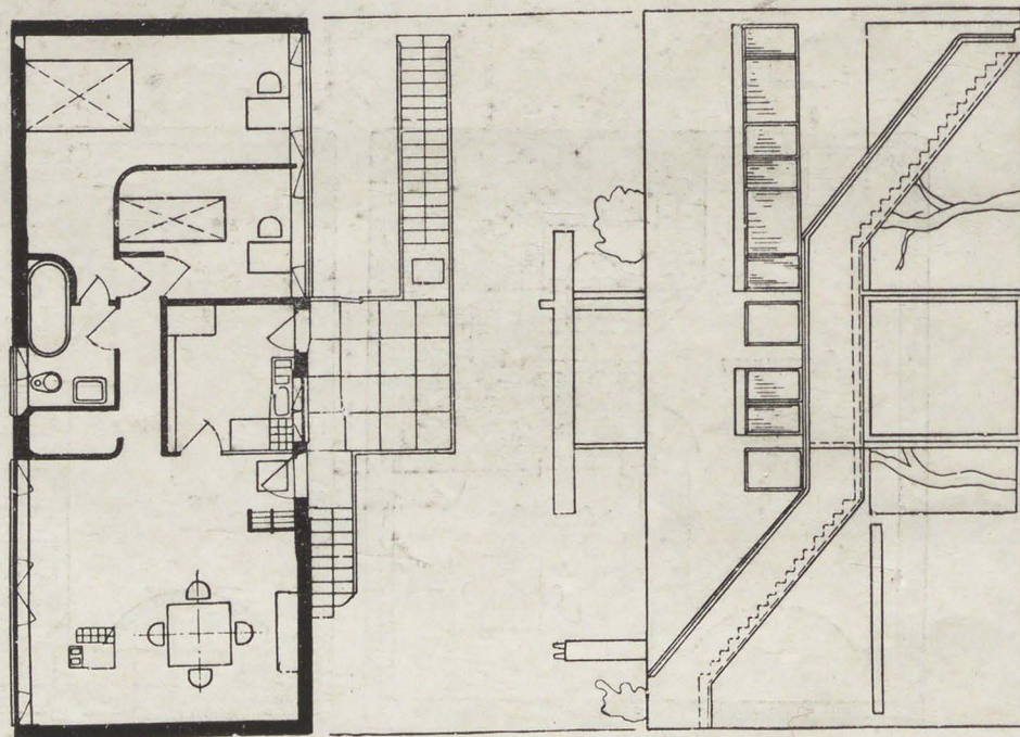
66. Жилой дом в поселке Пезак-Бордо. Корбюзье и Жаннере.
