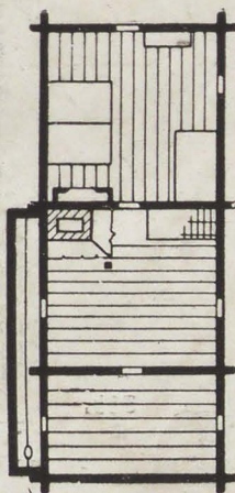
52 и 52 а, в, с. Старый шведский дом.
