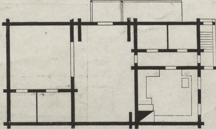
47. План вологодской избы.
