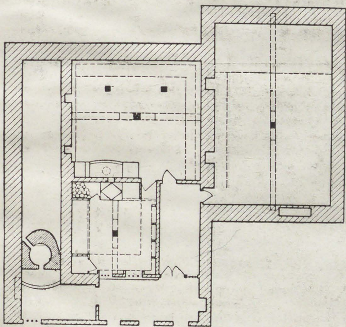
12. Старые дома в татарских деревнях Крыма. Планы. Разрезы. Фото фахверковой кладки.
