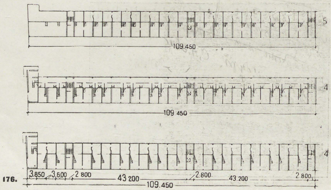
174, 175 и 176. Дом РЖСКТ „Рабочий“ в Саратове. Аксонометрия и планы этажей. С. А. Лисагор и Е. М. Попов
