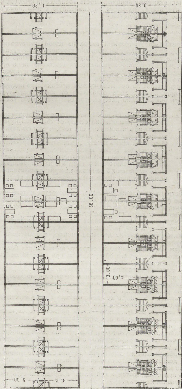
226. Гипрогор. Сектор Башкирских работ. Общежитие. Планы блоков трехкомнатных двухэтажных квартир.
