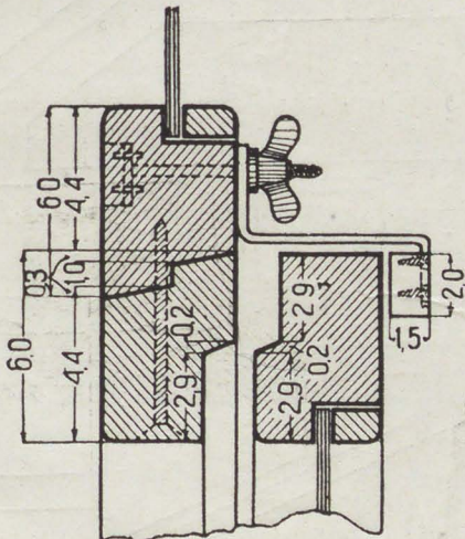
167. РЖСНТ „Показательное строительство“. Чертежи сдвижного окна М. О. Барщ, В. Н. Владимиров, И. Ф. Милинис, С. В. Орловский, А. Л. Пастернак и Л. С. Флавина
