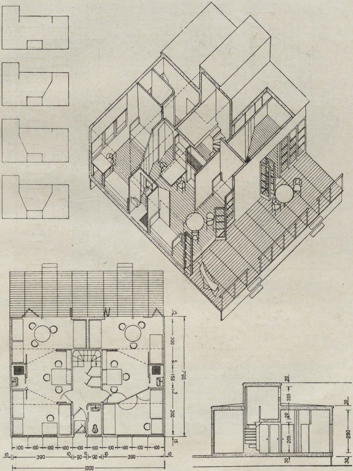
210. Госплан РСФСР. Секция соцрасселения. Общежитие с коридорной связью для семейных.
