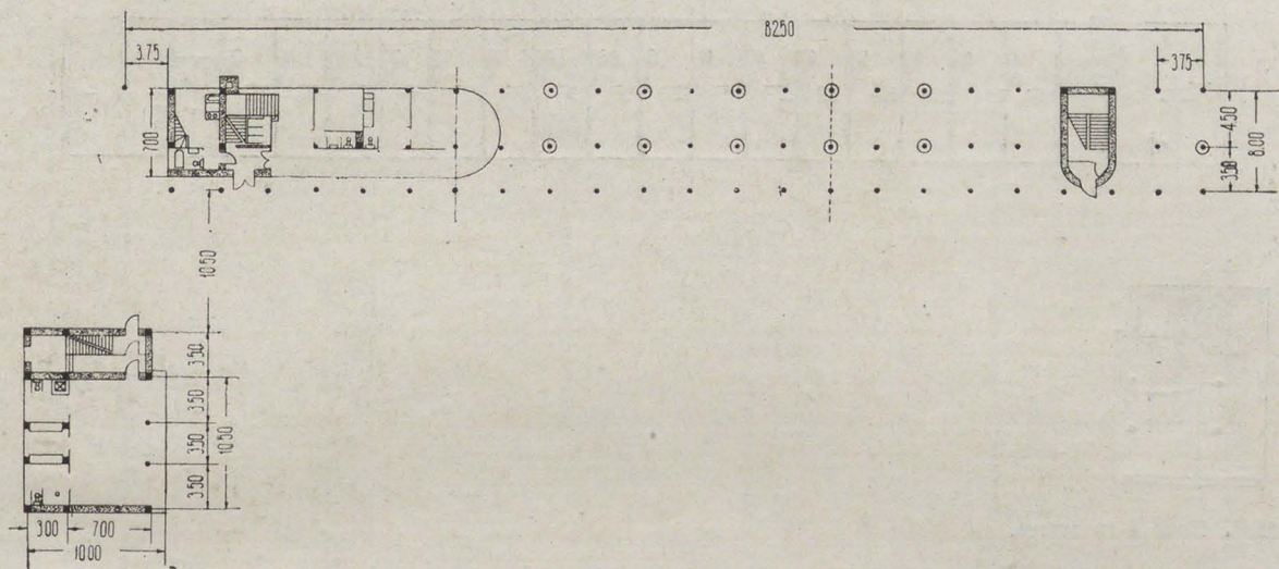
124. 2-й дом СНК. План 1-го этажа.
