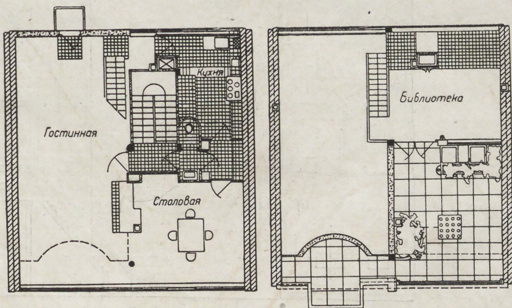
65. Норбюзье и Жаннере. Дом Нука в Париже.
