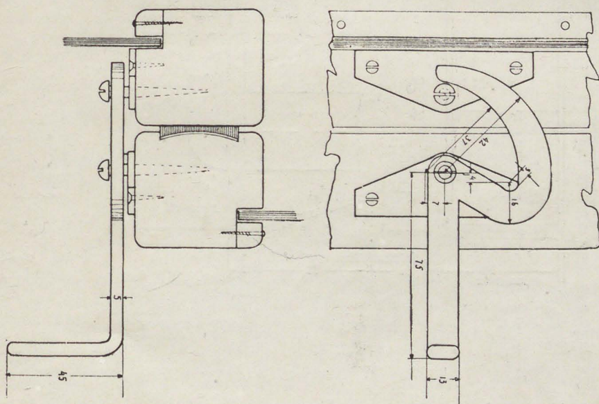
150. Рабоч. черт. для 2-го дома СНК. Прижим для сдвижного окна, М. Я. Гинзбург и И. Ф. Милинис
