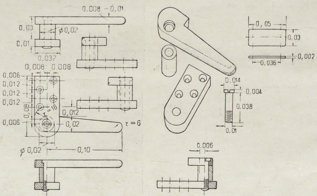
147—148. Рабоч. черт. для 2-го дома СНК. Прижим для сдвижного окна, М. Я. Гинзбург и И. Ф. Милинис
