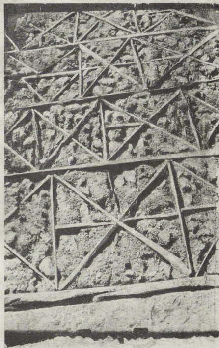
12. Старые дома в татарских деревнях Крыма. Планы. Разрезы. Фото фахверковой кладки.
