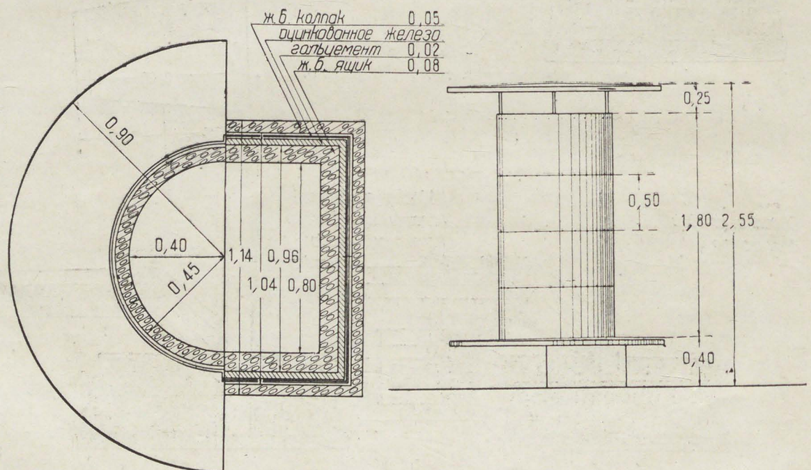
154. Рабоч. черт. для 2-го дома СНК. Детали гальцементной кровли. М. Я. Гинзбург и И. Ф. Милинис
