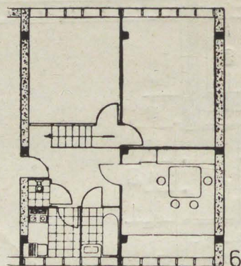
128. 2-й дом СНК. Планы квартиры—тип 2-Ф. 4-й, 5-й и 6-й этажи. М. Я. Гинзбург и И. Ф. Милинис
