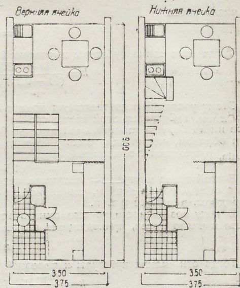
100. Типовой проект полустудионой квартиры—тип F. Разрез и планы. Стройком РСФСР
