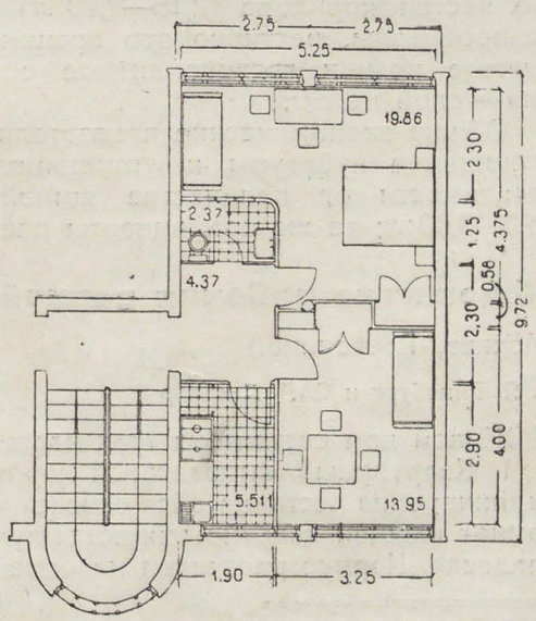
158. Дом Уралоблсвхоזה в Свердловске. Типовые ячейки. М. Я. Гинзбург и А. Л. Пастернат
