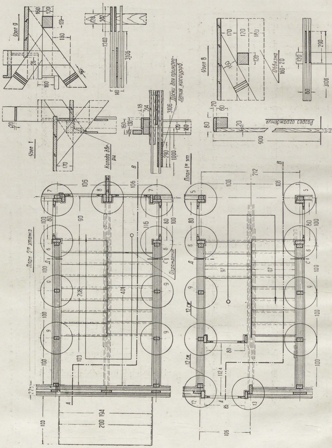
231. Гипрогор. Сектор Башкирских работ. Каркасно-соломитовые дома. Планы и детали лестницы
