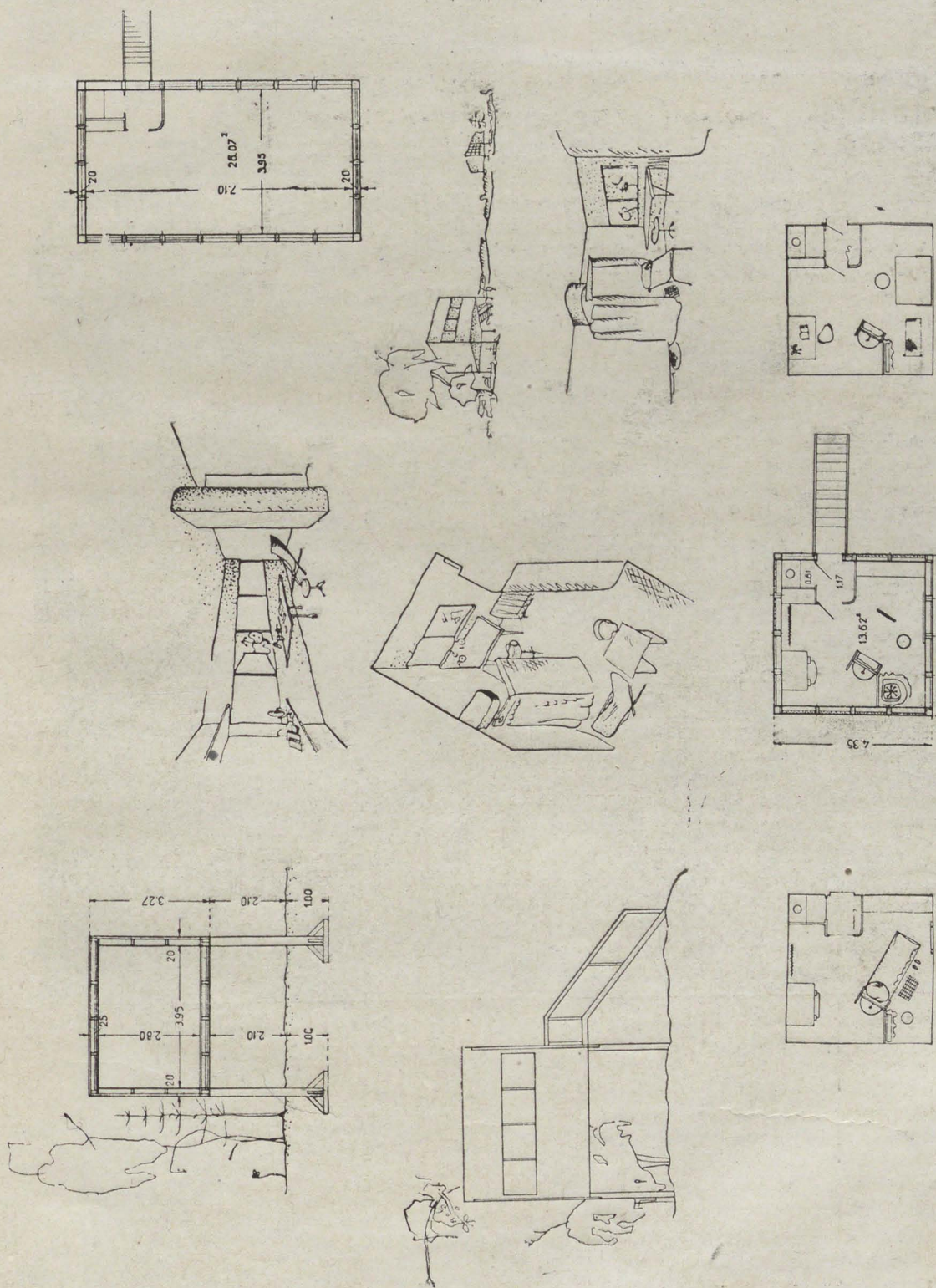
198. Проект Магнитогорья. Однокомнатная ячэйка. М. О. Барш, В. Н. Владимиров, М. Охитович, Н. Соколов, Н. П. Воротынцева
