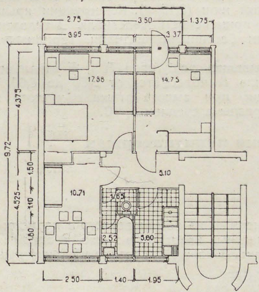
158. Дом Уралоблсвхоזה в Свердловске. Типовые ячейки. М. Я. Гинзбург и А. Л. Пастернат
