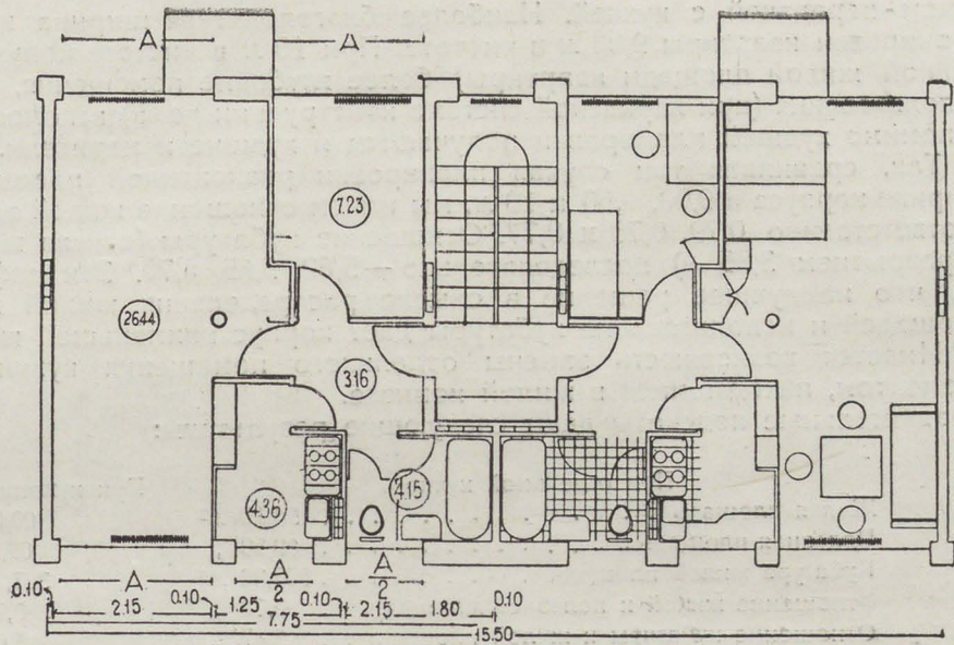
93. Типовой проект двухкомнатной квартиры. Стройком РСФСР
