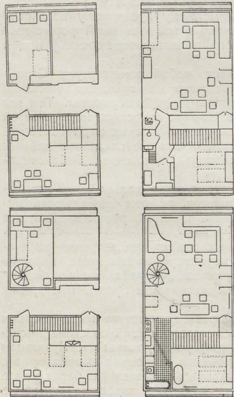
182, 183, 184. Дом-коммуна 1927 г. Манет разрез и планы М. Я. Гинзбург
