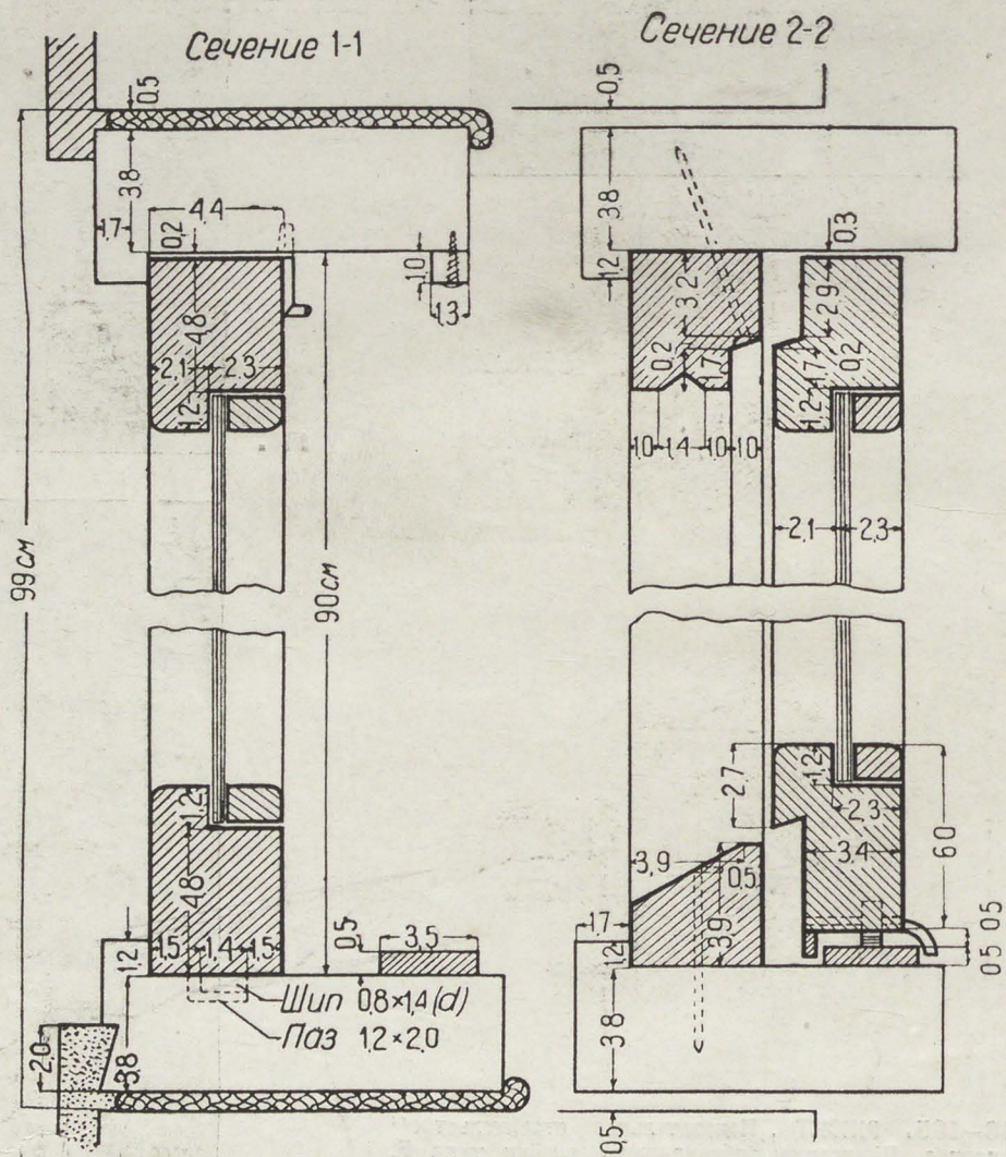
166. РЖСМТ „Показательное строительство“. Чертежи сдвижного окна М. О. Барщ, В. Н. Владимиров, И. Ф. Милинис, С. В. Орловский, А. Л. Пастернак и Л. С. Славина
