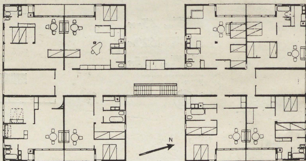
76. Жилой дом в Берлине арх. Радинг.
