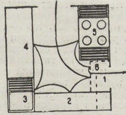
Рационализированная кухня 4,5 м 2
