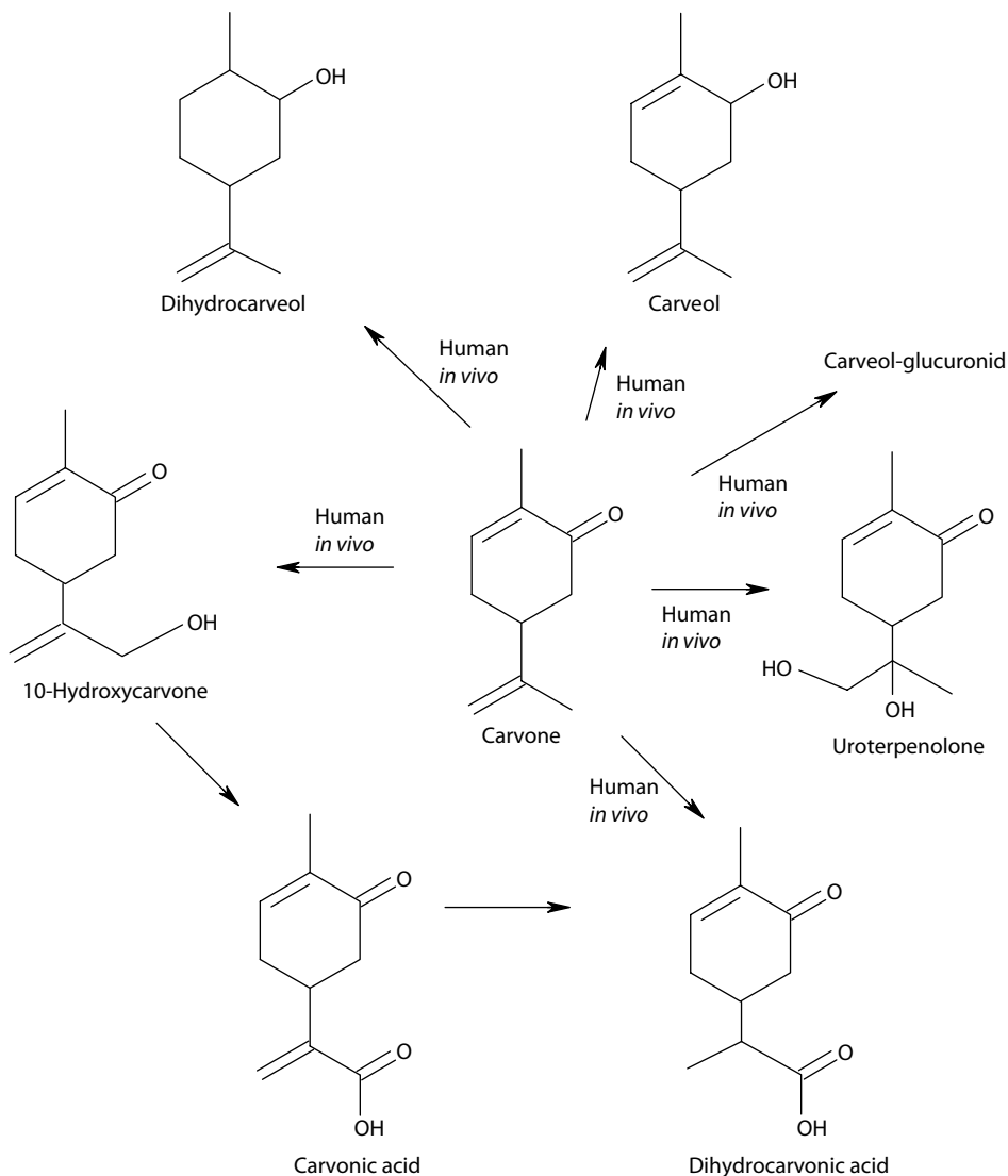
FIGURE 8.5 Proposed metabolic pathway of (R) -(-)- and (S) -(+)-carvone in healthy volunteers. (Adapted from Engel, W., 2001. J. Agric. Food Chem. , 49: 4069–4075; Jahrman, R., 2007. Metabolismus von Monoterpenen und Sesquiterpenen in Mensch und Säugetier: Bedeutung für die pharmazeutische Praxis . MPharm. diploma thesis, University of Vienna, Austria.)
