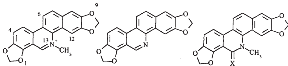
sanguinarine
