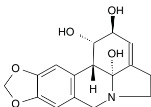
Lycorine
