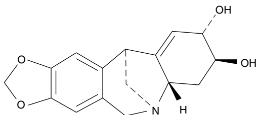
68 pancracine
