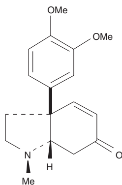
82 mesembrenone ( Scelletium )
