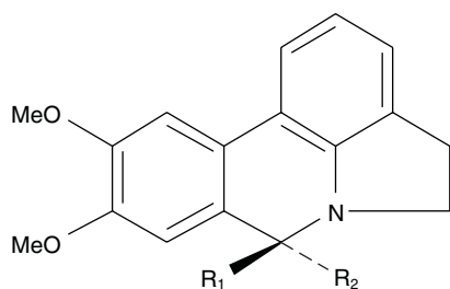
18 assoanine
