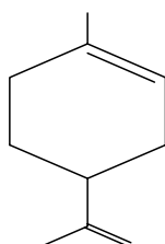
imonene
