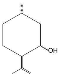
neoiso(pulegol)
