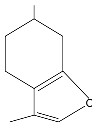
menthofuran
