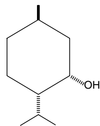
neomenthol
