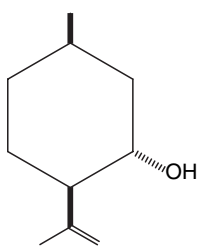
iso(iso)pulegol
