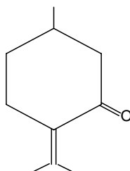
pulegone
