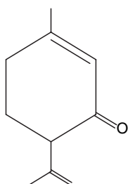
isopiperitenone
