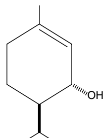
trans -piperitol
