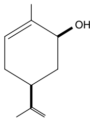
cis-carveol
