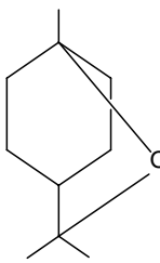
1,8-cineole
