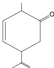
spicatonone
