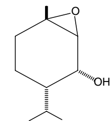
1,2-epoxyneomenthol
