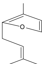
rosefuran
