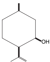
neoiso(iso)pulegol
