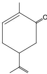
carvone
