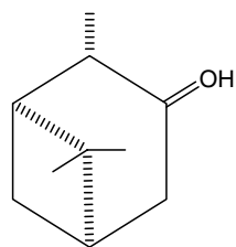
isopinocampone
