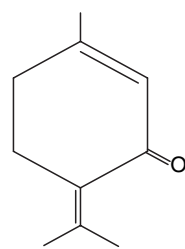
piperitenone
