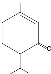
piperitone
