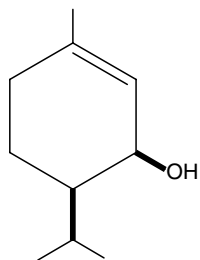
cis -piperitol
