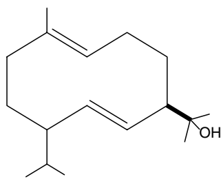
elemol
