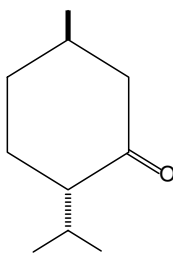
menthone
