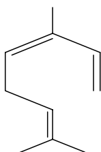
(Z)-β-ocimene
