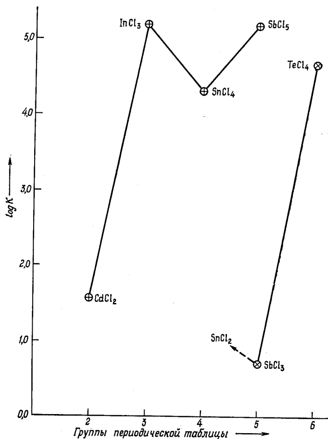
Рис. 10. Константы образования хлоро-комплексов из (C_6H_5)_3CCl и некоторых хлоридов в ацетонитриле.
