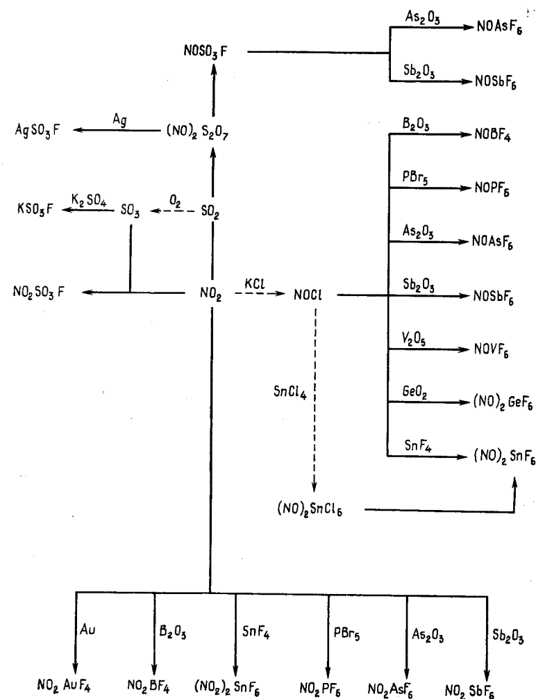
Рис. 9. Схематическое представление некоторых реакций в жидком \text{BrF}_3 .
