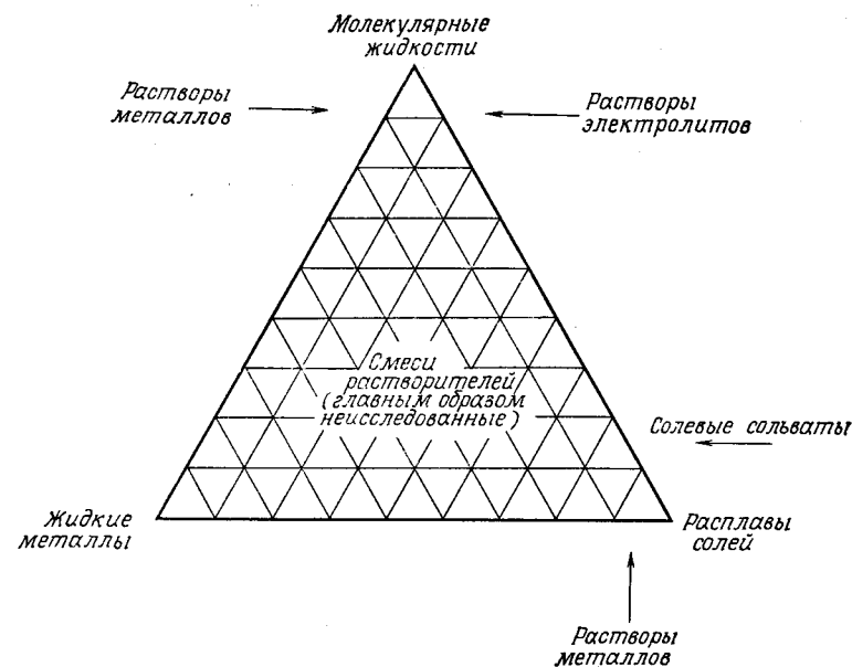
Рис. 1. Типы растворителей.
