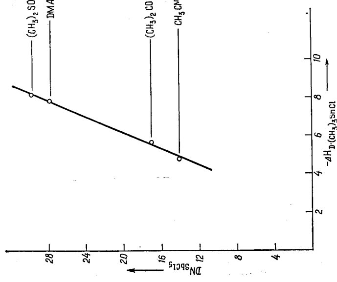
Р и с. 5. Соотношение между \text{DN} \cdot \text{SbCl}_5 и -\Delta H_{D \cdot (\text{CH}_3)_3\text{SnCl}} для различных донорных растворителей D.
