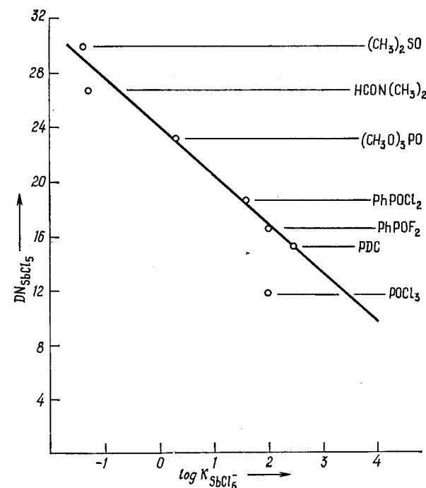
Рис. 8. График зависимости \log K_{SbCl_6^-} от DN_{SbCl_5} в различных растворителях.
