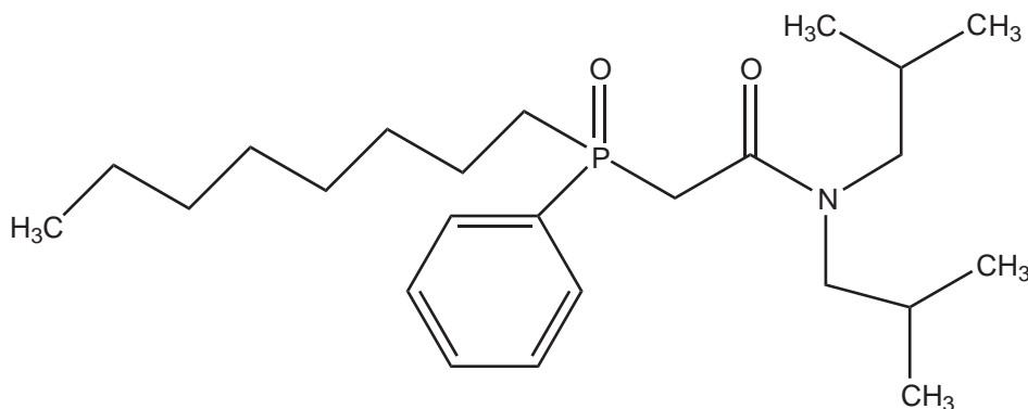
Figure 26 CMPO.
