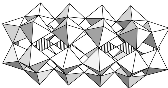
Figure 17 [(P_2O_7)_2Mo_{30}O_{90}]^{8-} .
