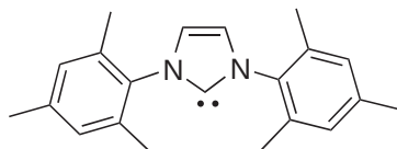
L25
