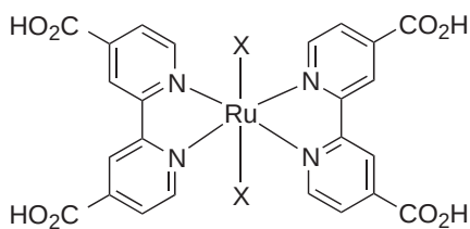
(35) X = Cl -
