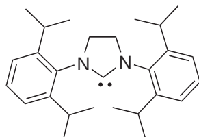
L27
