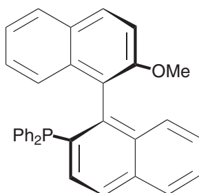
( S )-MeO-MOP ( 22 )
