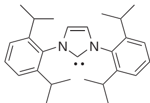
L24
