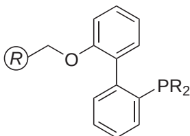
L29
