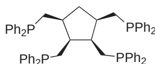
L18
