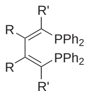
L17
