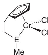
E = O, (93);
