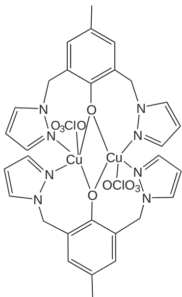
\{[Cu(L)](OCIO_3)\}_2 (307)
