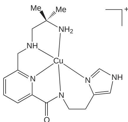
[(L)Cu][ClO 4 ] (459)
