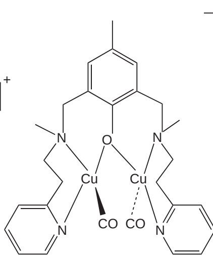
[(L)Cu_2(CO)_2][PF_6] ( 731 )
