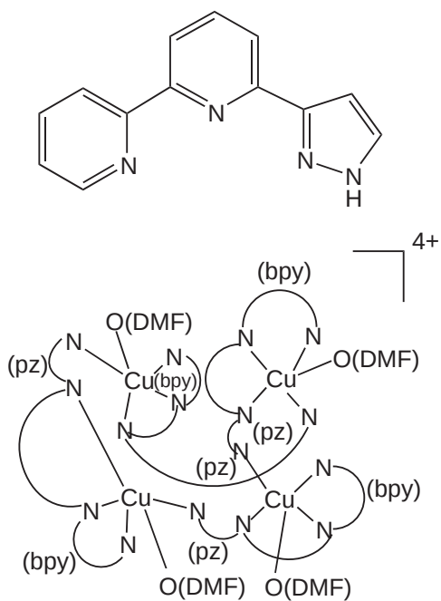
[(\text{L})_4\text{Cu}_4(\text{DMF})_4][\text{PF}_6]_4 ( 602 )
