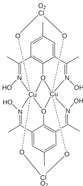
[(H_2L)_2Cu_2(OCIO_3)_2] (374)
