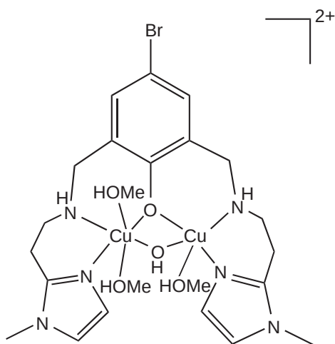
[(L)Cu_2(OH)(MeOH)_2][BF_4]_2 ( 367 )
