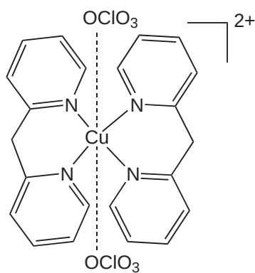
[(L)_2Cu(OCIO_3)_2] ( 201 )
