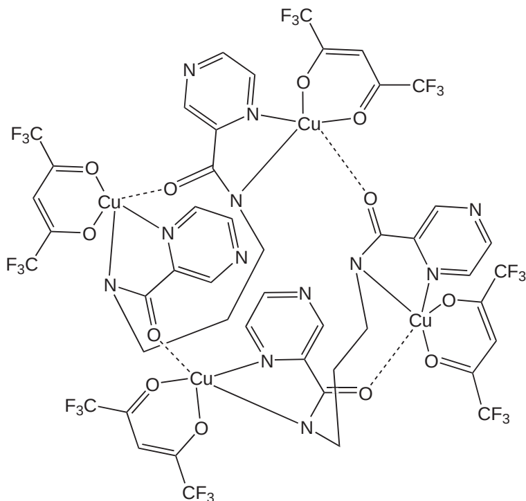
[(L)Cu(L')_2Cu]_2 ( 490 )
