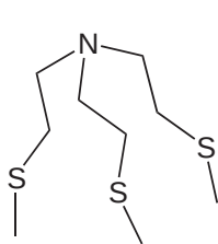
[(\text{L})\text{CuBr}][\text{ClO}_4] ( 426 )
