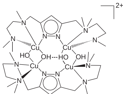
[(L)_2Cu_4(OH)_4][PF_6]_2 ( 147 )
