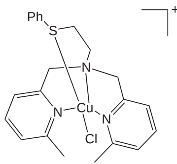
[(\text{L})\text{CuCl}][\text{ClO}_4] ( 429 )
