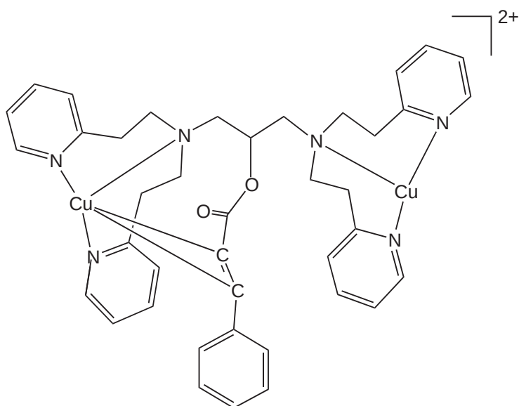
[Cu_2(L)][PF_6]_2 ( 732 )
