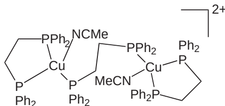
[(L)Cu(MeCN)]_2[ClO_4]_2 ( 768 )
