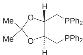
(85) S,S -DIOP
