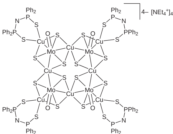
( 193 ): n_2 = -1.7 \cdot 10^{-10} \text{ cm}^2 \text{ W}^{-1} \text{ M}^{-1} , \alpha_2 = 1.0 \cdot 10^{-5} \text{ cm W}^{-1} \text{ M}^{-1} (DMF) 512
