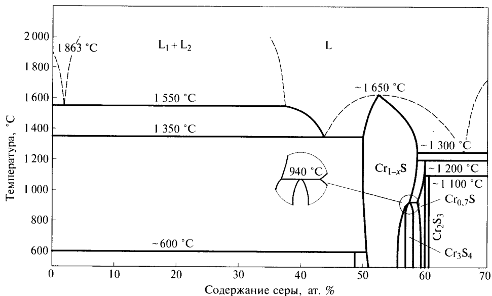
Рис. 4.33. Фазовая диаграмма системы хром—серы (темным показаны области гомогенности сульфидов \text{Cr}_{1-x}\text{S} , \text{Cr}_{0.7}\text{S} , \text{Cr}_3\text{S}_4 ; фазы \text{Cr}_7\text{S}_8 и \text{Cr}_5\text{S}_6 образуются при температуре 320 и 325 °C соответственно)
