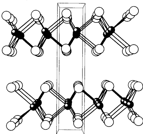
Рис. 4.34. Кристаллическая структура \text{MoS}_2 : a — общий вид; б, в — проекции вдоль координатных плоскостей
