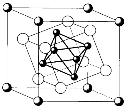
Рис. 4.35. Структура фазы Шевреля \text{PbMo}_6\text{S}_8
