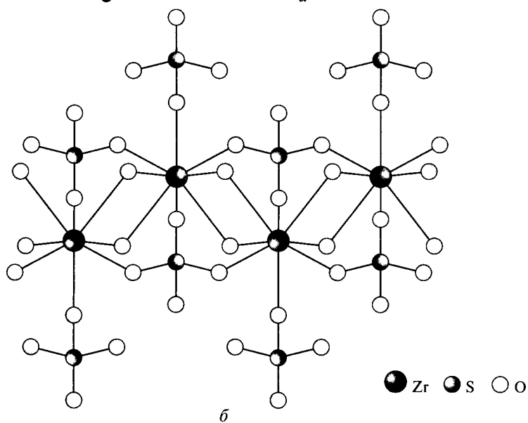
Рис. 2.13. Оксо- и гидросульфаты титана и циркония: a — сульфат титанила \text{TiOSO}_4 \cdot \text{H}_2\text{O} ; б — гидросульфат циркония \text{Zr}(\text{OH})_2\text{SO}_4 (атомы водорода не показаны)
