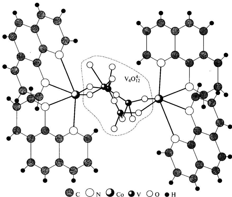
Рис. 3.21. Строение комплекса \text{Co}_2(\text{phen})_4\text{V}_4\text{O}_{12}
