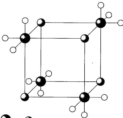
Рис. 4.36. Структура кластера состава [\text{Mo}_4\text{S}_4(\text{H}_2\text{O})_{12}]^{n+}
