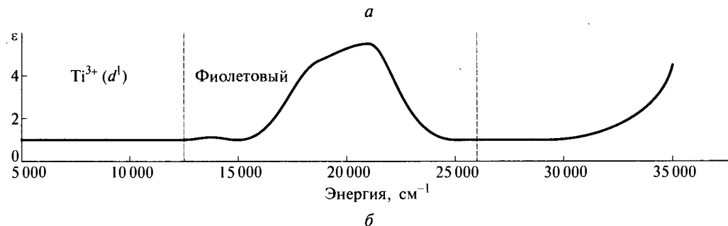
Рис. 1.35. Электромагнитная шкала (а); электронный спектр иона [\text{Ti}(\text{H}_2\text{O})_6]^{3+} (б); расщепление термина {}^2D (в) (переход электрона, вызывающий окраску, показан стрелкой)
