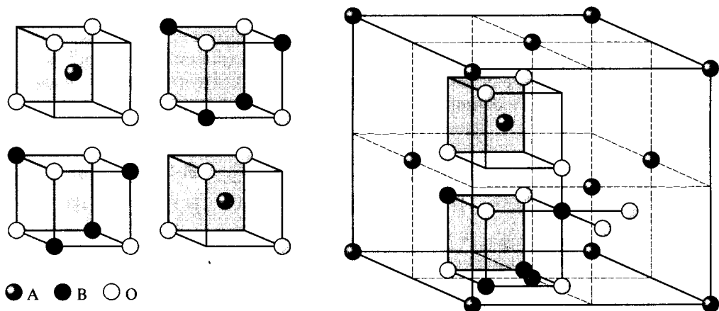
Рис. 1.21. Структура шпинели
