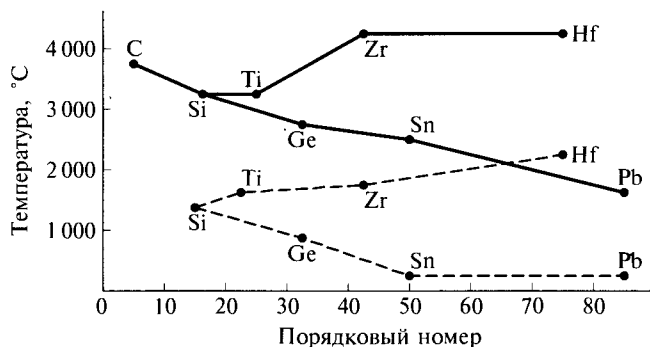
Рис. 2.5. Зависимость температуры плавления (пунктирные линии) и температуры кипения (сплошные линии) простых веществ 4-й и 14-й групп от порядкового номера
