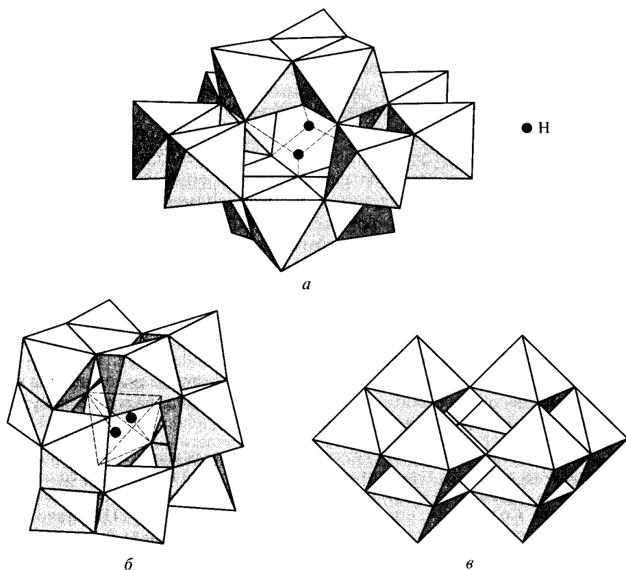
Рис. 4.22. Строение вольфраматов:
