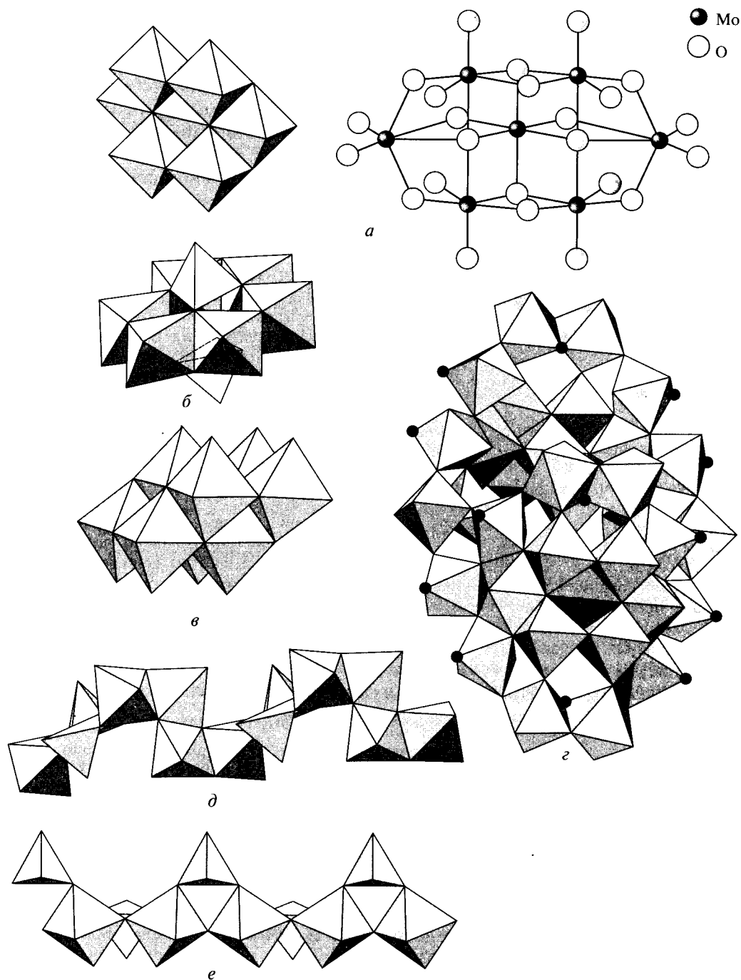
Рис. 4.21. Разнообразие изополимолибдатов:
