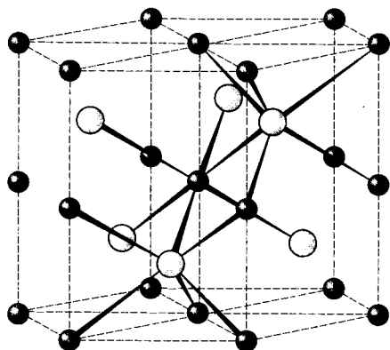
NiAs
