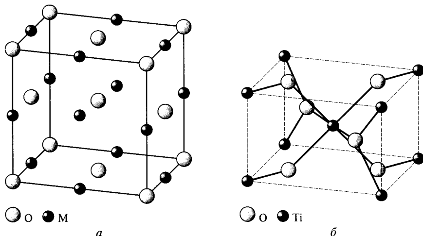
Рис. 1.16. Структура хлорида натрия (галита) (а) и рутила (б)
