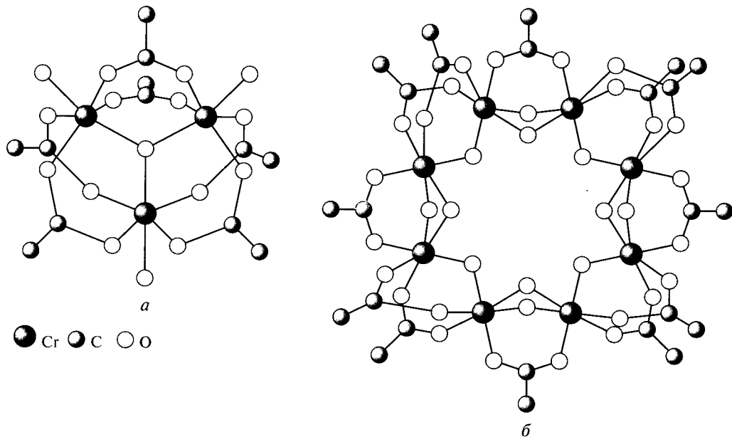
Рис. 4.12. Оксо- и гидроксоацетаты хрома(III):
