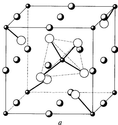
Рис. 3.31. Строение тиованадатов: а — \text{Ti}_3\text{VS}_4 ; б — цепи из октаэдров [\text{VS}_6] в \text{BaVS}_3
