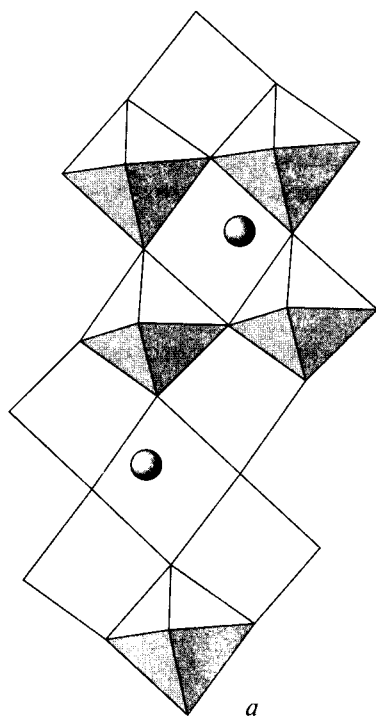
Рис. 3.22. Структура ванадиевой бронзы (а) (атомы Na расположены между слоями из пирамид [VO_5] в структуре V_2O_5 ); фазовая диаграмма системы V_2O_5 - Na_2O (б) (изотерма при 426 °С показывает полиморфный переход в Na_4V_2O_7 )
