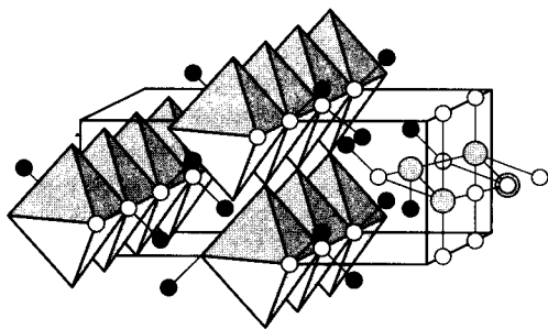
Рис. 3.11. Строение оксогидроксида \text{VO}(\text{OH})_2
