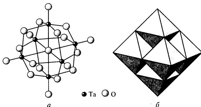
Рис. 1.22. Структура аниона гексатанталата [Ta_6O_{19}]^{8-} в виде атомов (а) и в форме полиэдров (б)
