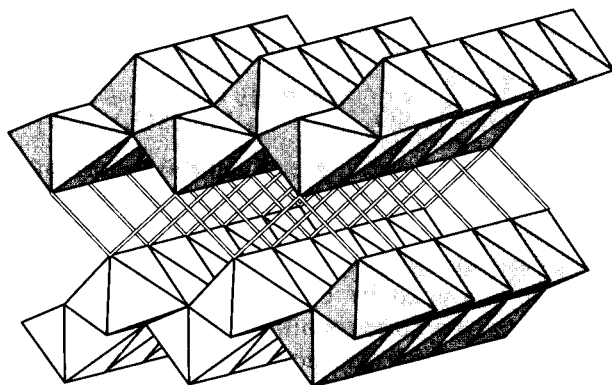
Рис. 5.23. Строение оксигидроксидов \alpha -MnOOH (a) и \gamma -MnOOH (б)
