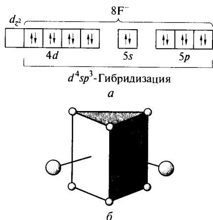
Рис. 2.2. Схема образования комплекса [\text{ZrF}_8]^{4-} по методу валентных связей (а) и его строение (б)
