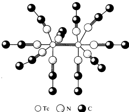
Рис. 5.22. Строение комплекса [Tc_2(CH_3CN)_{10}]^{4+} (атомы водорода не показаны)
