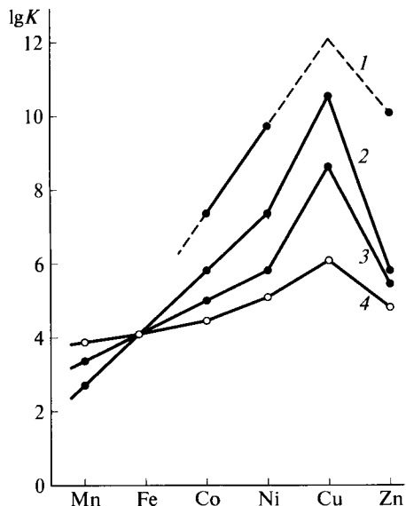
Рис. 1.34. Зависимость константы устойчивости комплекса состава [M(H_2O)_5L]^{(2-x)+} от природы 3d -металлов для ряда лигандов (L):
