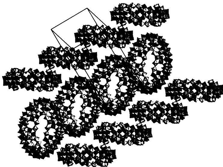
Рис. 4.26. Молибденовые «сѣни»:
