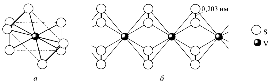
Рис. 3.32. Строение VS_4 :
