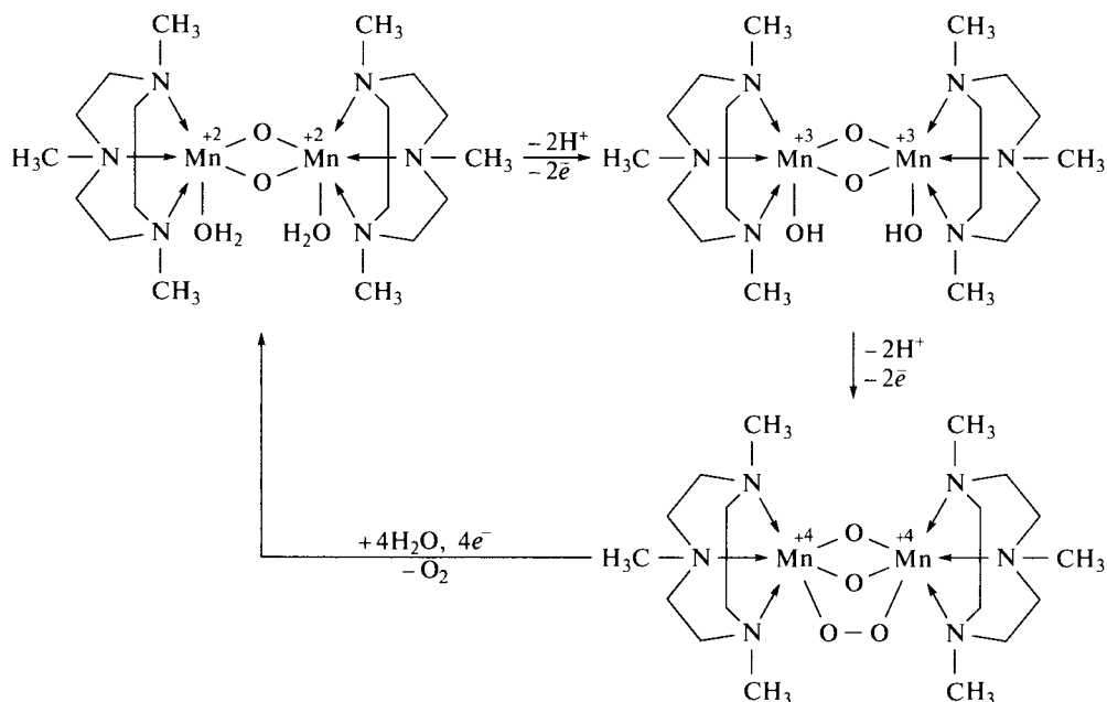
Рис. 5.29. Предполагаемый механизм окисления воды активным центром марганецсодержащего олигопротеинового комплекса (показан на модельном соединении с лигандом 1,4,7-триметил-1,4,7-триазациклононаном)
