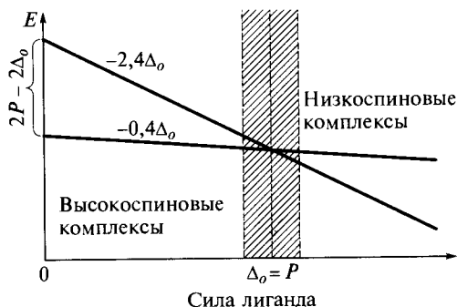
Рис. 1.27. Изменение энергии стабилизации кристаллическим полем в зависимости от силы лиганда для высокоспиновых и низкоспиновых комплексов с конфигурацией иона металла d^6 (область, в которой возможно существование обоих состояний, заштрихована)
