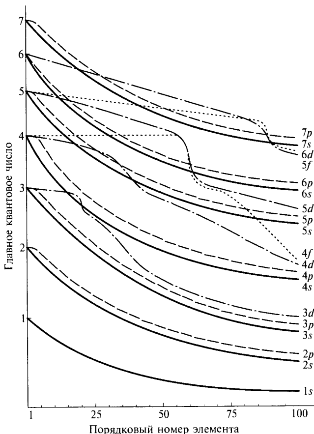
Рис. 1.2. Зависимость энергии атомных орбиталей от порядкового номера элемента
