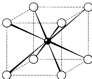
CsCl
