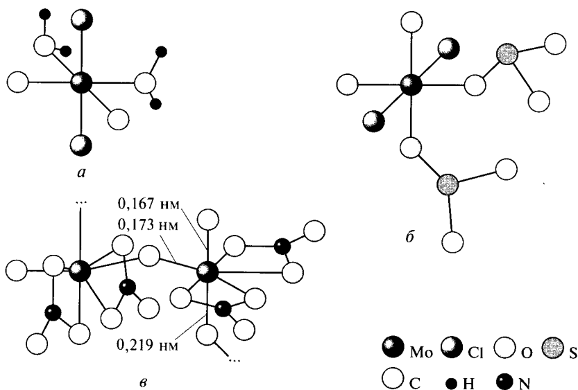
Рис. 4.23. Строение комплексов:
