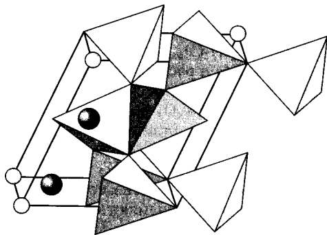
Рис. 5.20. Строение \text{K}_2\text{Mn}_2\text{O}_3
