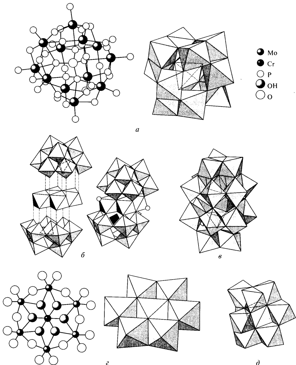
Рис. 4.25. Строение гетерополианионов:
