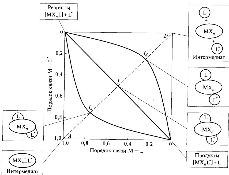
Рис. 1.40. Возможные механизмы реакции замещения MX_nL + L^* \rightarrow MX_nL^* + L , типы интермедиатов и переходных состояний:
