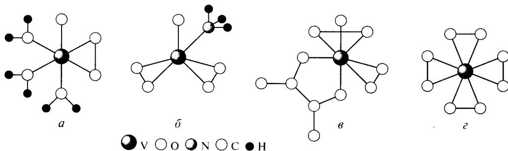
Рис. 3.27. Строение ионов:
