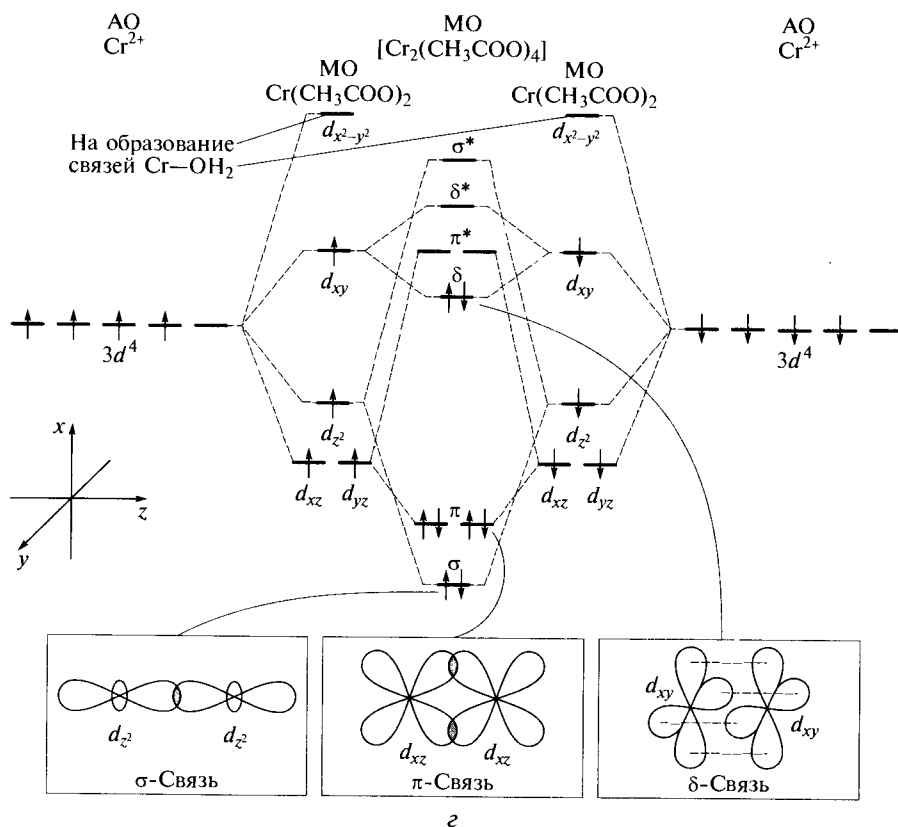
Рис. 4.7. (Окончание)
