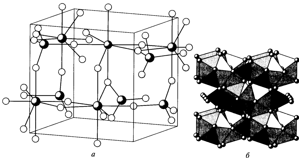
Рис. 2.4. Строение циркона:
