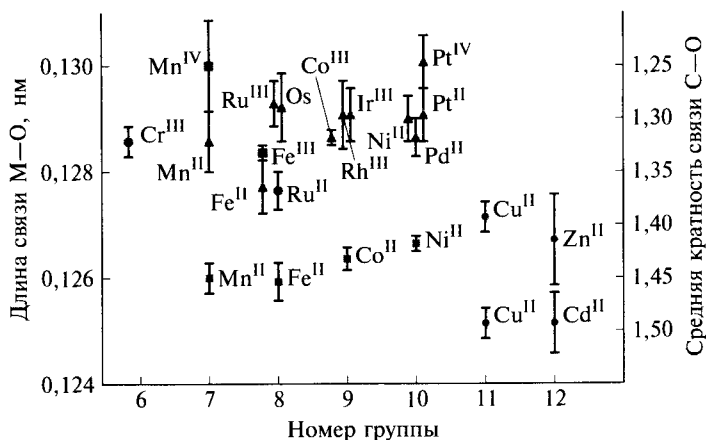
Рис. 1.7. Зависимость длины связи металл — лиганд и кратности связи углерод — кислород в карбоксилатах переходных металлов от номера группы (точки ▲ — низкоспиновые, ■ — высокоспиновые комплексы)
