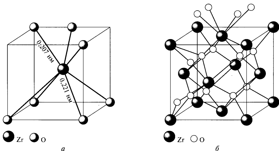
Рис. 2.7. Строение оксида ZrO 2 : a — моноклинный (бадделейт); б — кубический
