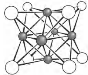
[Mo 6 Cl 8 ] 4+
