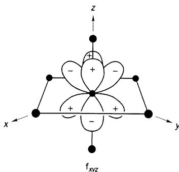
f_{xyz}
