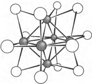
[Ta 6 Cl 12 ] 2+
