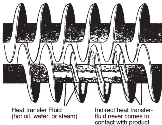
FIG. 18-52 Holo-Flite Processor. (Denver Sala.)
