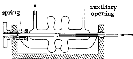
Fig. 32. Bodenstein valve.
