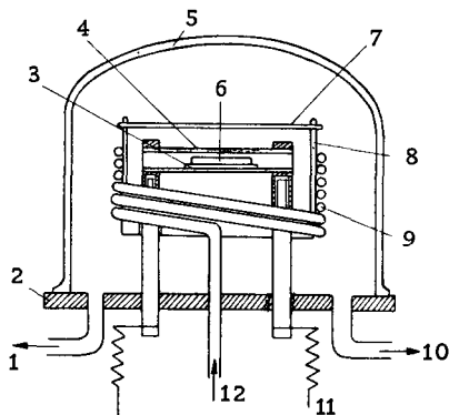
Fig. 12. Tungsten furnace.
