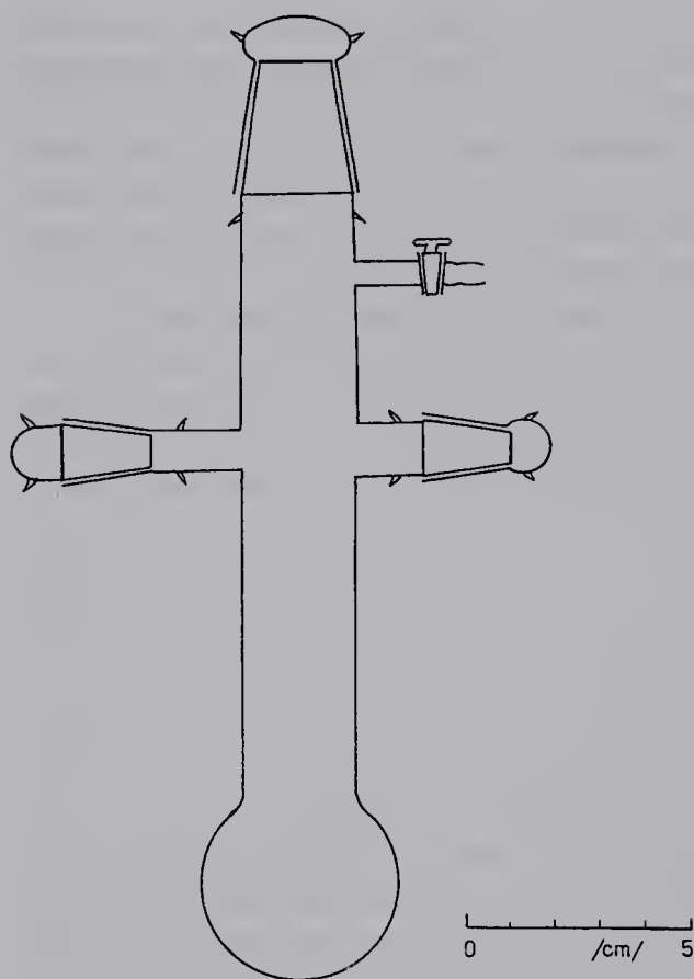
Fig. 3.28-1 Sublimation apparatus.
