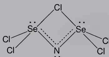
\text{Se}^{\text{IV}}_2\text{NCl}_5
