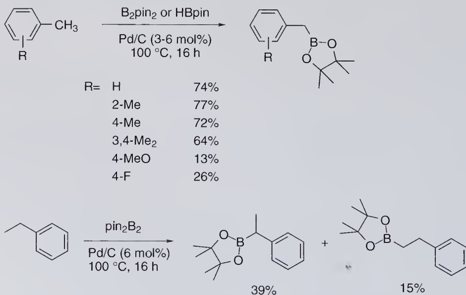
Scheme 2.15 Benzylic C–H borylation.
