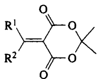
(8)
