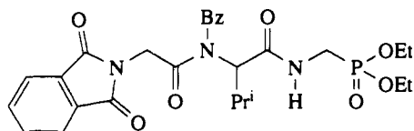
(113)
