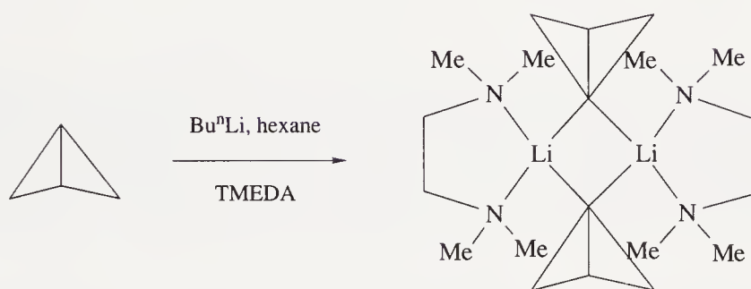
(47)
