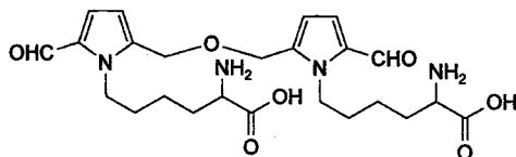
Bis-pyrraline
