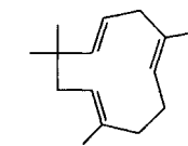
Humulene (XLIV)
