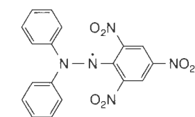
Diphenylpicrylhydrazyl (DPPH)
