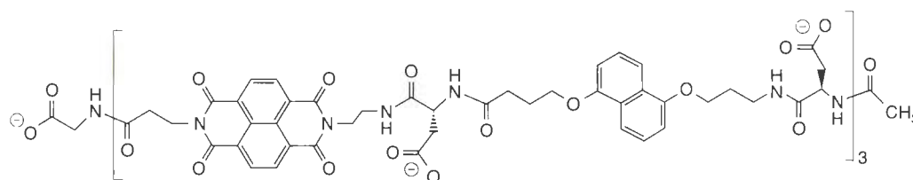
Linear aedamer
