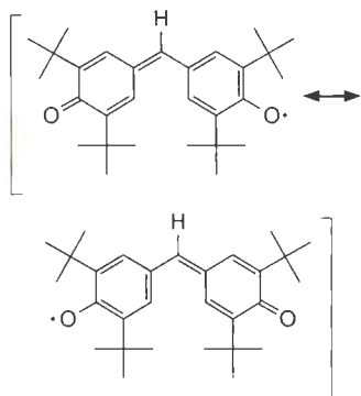
Galvinoxyl
