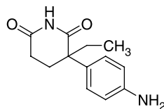
15 , Aminoglutethimide
