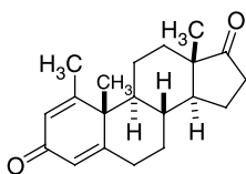
14 , Atamestane
