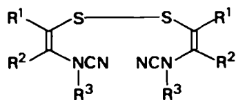
(102)
