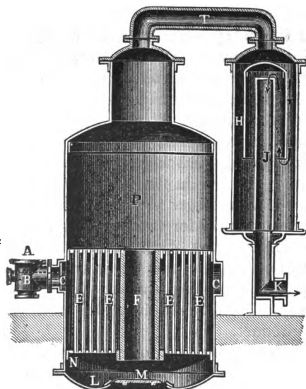
FIG. 45.—Vacuum-pan.
