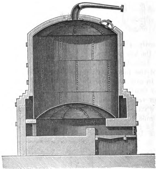
FIG. 58A.—Tar still.
