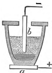
FIG. 43.—Formation of Calcium carbide.
