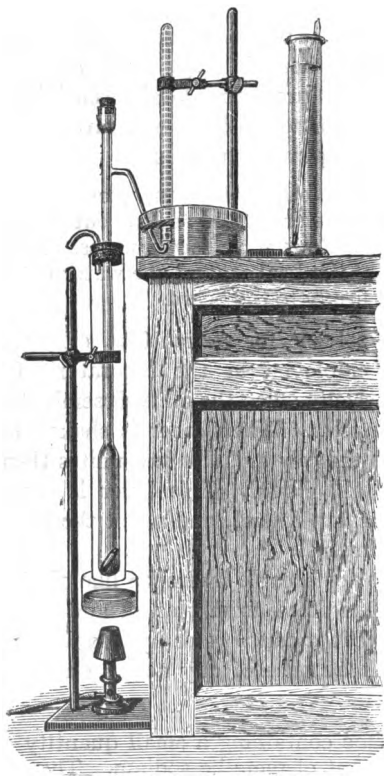
FIG. 21.—The Victor Meyer vapour density apparatus.
