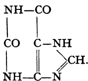
Xanthine.
