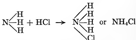
Ammonia
