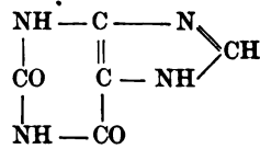
Xanthine
