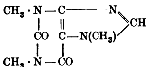
Caffeine
