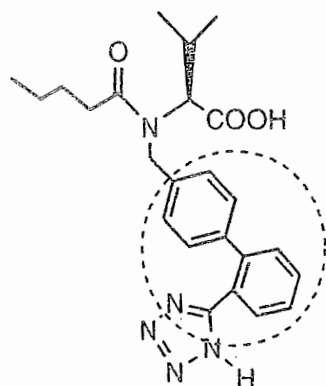
Valsartan
