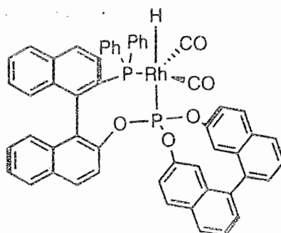
HRh(CO) 2 (R,S)-BINAPHOS
