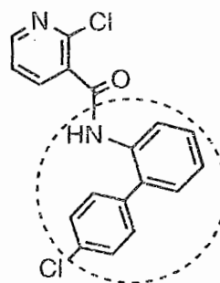
Boscalid
