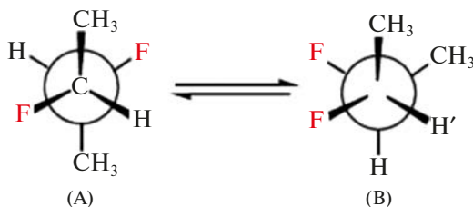
Рис. 8.9. Два конформера эритро -2,3-дифторобутана (а) и (б) обладают равной устойчивостью
