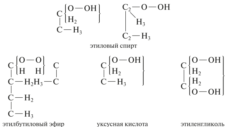
Схема 1.3. Химические формулы А. Купера
