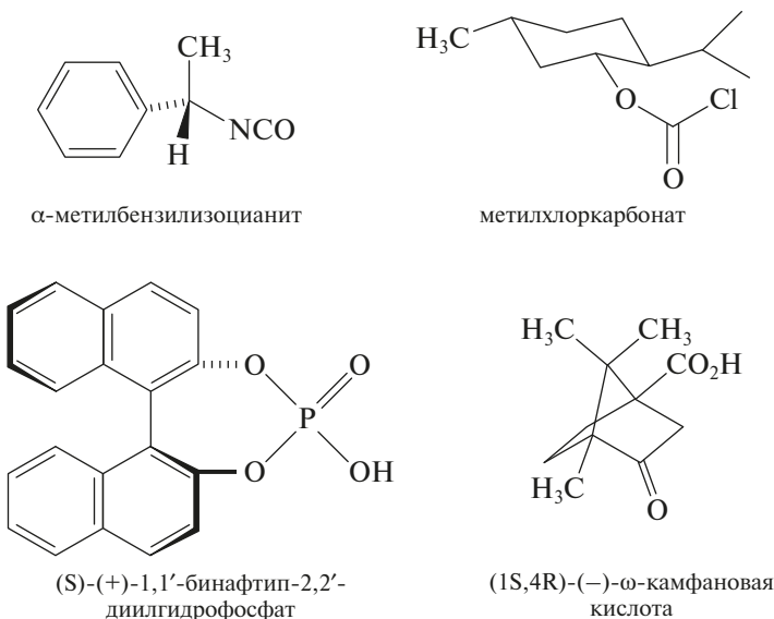
Рис. 7.37 (окончание). Хиральные расщепляющие реагенты
