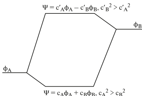
Рис. 3.18. Вид МО при образовании гетероядерной двухатомной молекулы
