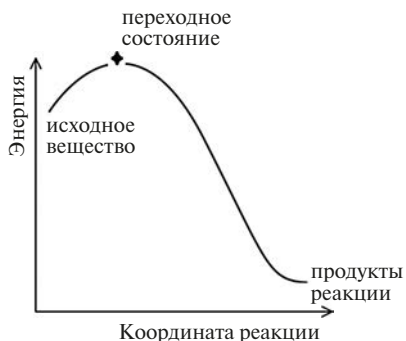
Рис. 9.1. Профиль изменения энергии системы в элементарной стадии реакции
