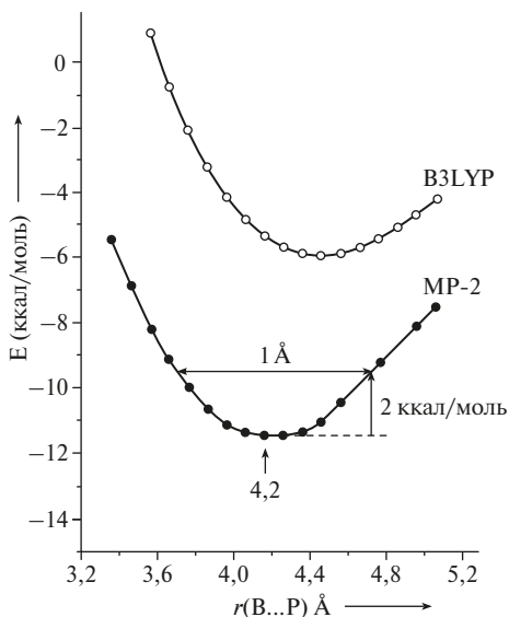
Рис. 5.22. Зависимость энергии «рыхлой лыюисовой пары» B(C_6F_5)_3 + P(tBu)_3 от расстояния Р---В по данным расчетов двумя методами
