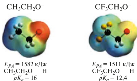
Рис. 6.4. Сравнение карт МЭП анионов, а также значений E_{pA} и pK_a этанола и 2,2,2-трифторэтанола показывает, что 2,2,2-трифторэтанол — более сильная кислота
