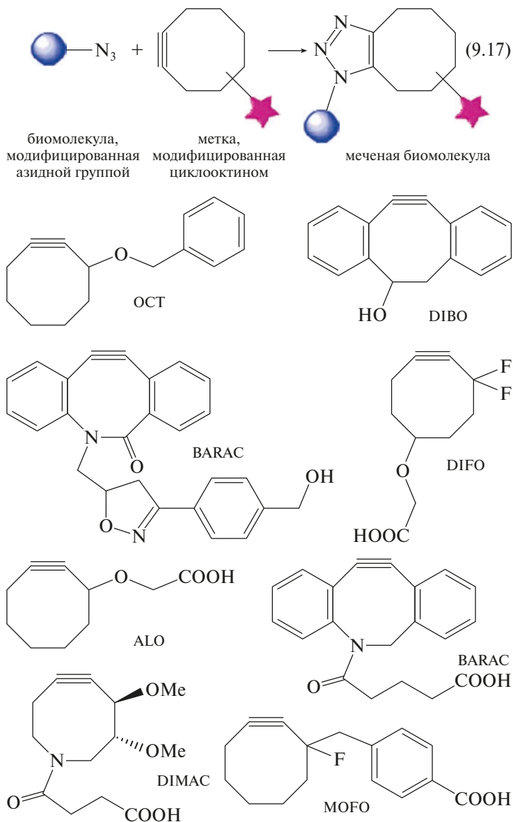
Рис. 9.13. Производные циклооктина, применяемые в реакции некатали- тического [3+2]-циклоприсоединения с азидом
