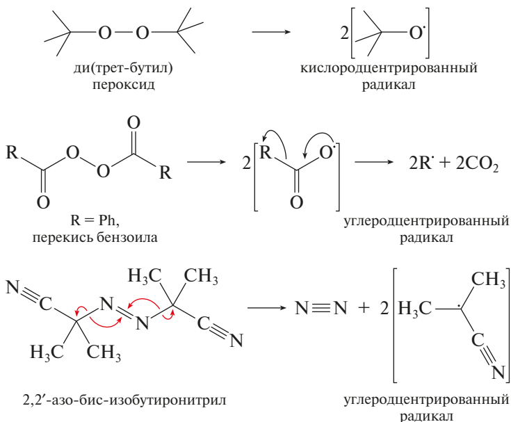
Рис. 9.5. Иницирование цепи в радикальных реакциях можно осуществить реакциями термолитического и фотолизического разложения пероксидов и азосоединений
