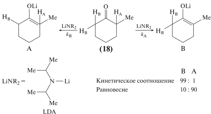
Рис. 6.21. Кинетический и термодинамический контроль в реакции депротонирования 2-метилциклогексанола ( 29 )
