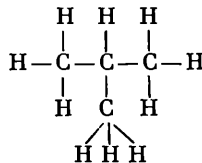
Isobutane
