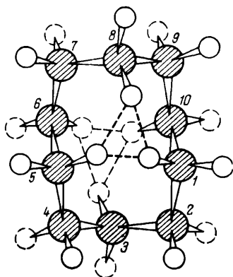
Fig. 6.3. Cyclodecane.
