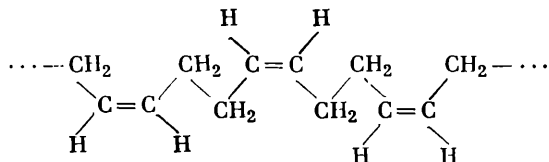
cis -Polybutadiene
