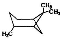
Pinocamphane
