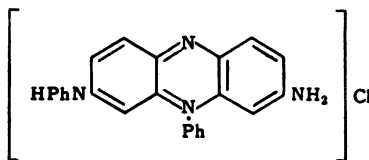
Pseudomauveine
