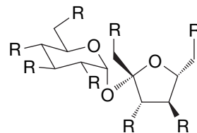
Olestra
