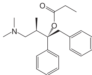
Darvon
