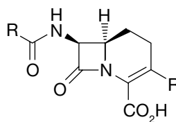
Cephalosporins
