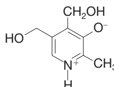
Pyridoxine
