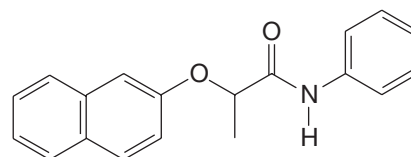
Naproanilide
