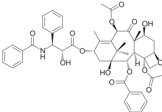
Paclitaxel (Taxol)
