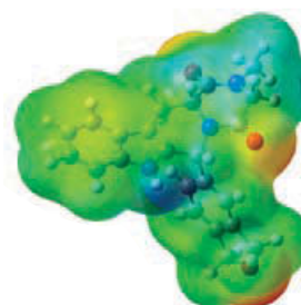
Cialis
