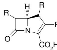
Carbapenem
