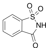
Saccharin
