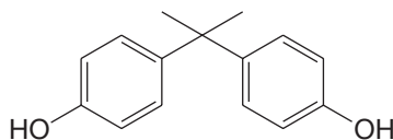
Bisphenol A
