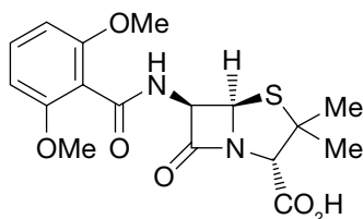
Methicillin
