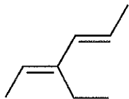
(2 E ,4 E )-3-ethylhexa-2,4-diene
