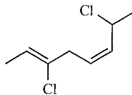
(2Z,5Z)-3,7-dichloroocta-2,5-diene
