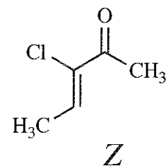
( Z )-3-chloropent-3-en-2-one
