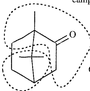
camphor
