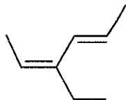
(2 Z ,4 E )-
