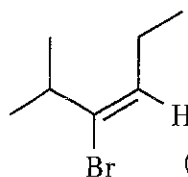
(2 Z ,4 E )-
