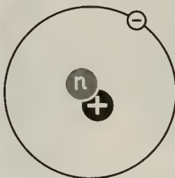
^2\text{H} ("DEUTERIUM")
