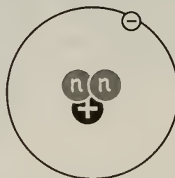
^3\text{H} ("TRITIUM")
