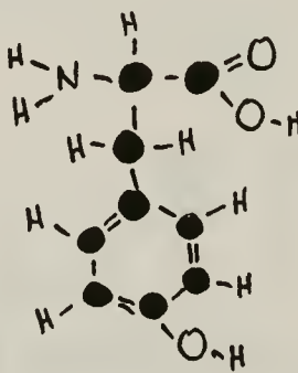
TYROSINE
