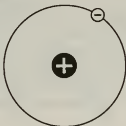
^1\text{H}
