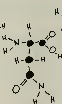
ASPARAGINE
