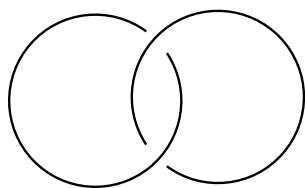
a [2]catenane
