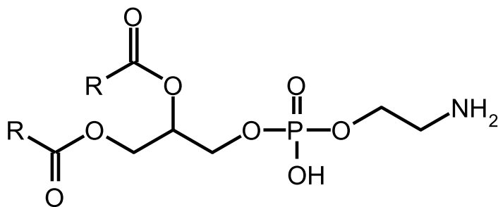
2-aminoethyl phosphatidates
