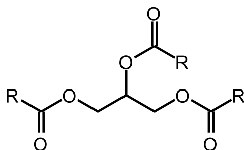
(a triglyceride)
