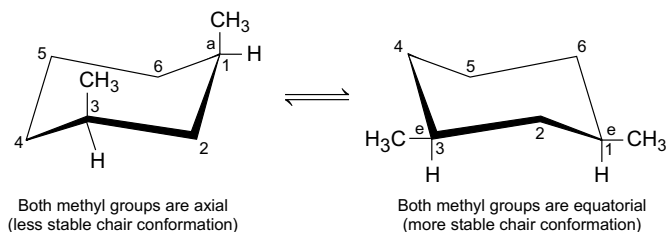
Fig. 2.24 Cis -1,3-Dimethylcyclohexane
