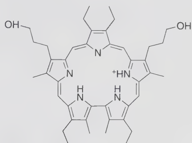
sapphyrin 33
