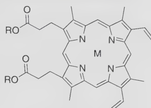
protoporphyrin IX
