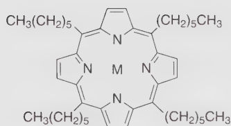
metal tetrahexylporphyrins 5
