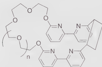
58a n=1 Y. 41%
