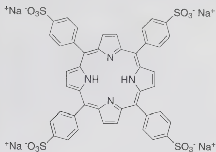
tetrakis(4-sulfonatophenyl)porphyrin 32
