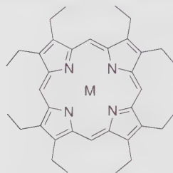
metal octaethylporphyrins 4
