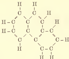
Anthracene.
