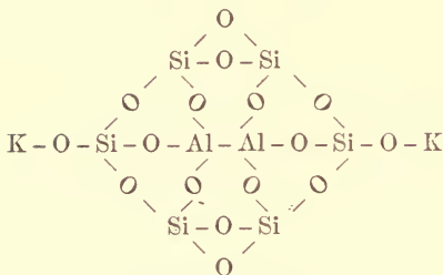
Feldspar (Orthoclase).
