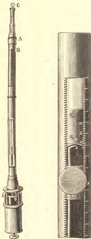
FIG. 5.—Barometer.
