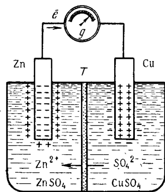
Рис. 1. Схема гальванического элемента
