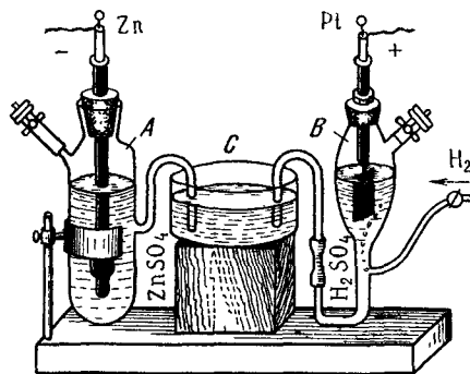
Рис. 2. Определение нормального потенциала металла
