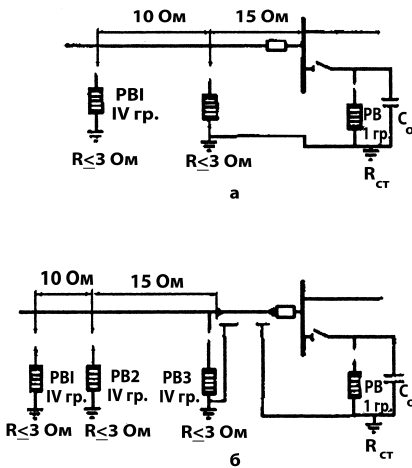
Рис. 4.2.21. Схемы защиты электродвигателей мощностью до 3 МВт при подходе ВЛ на деревянных опорах
