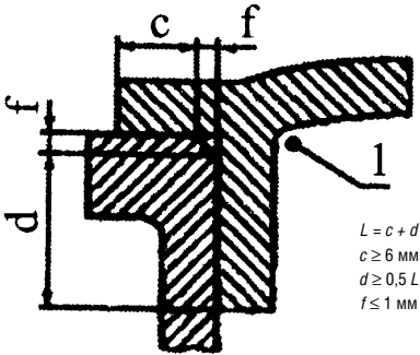
Рис. П5.8. Плоскоцилиндрическое взрывонепроницаемое соединение
