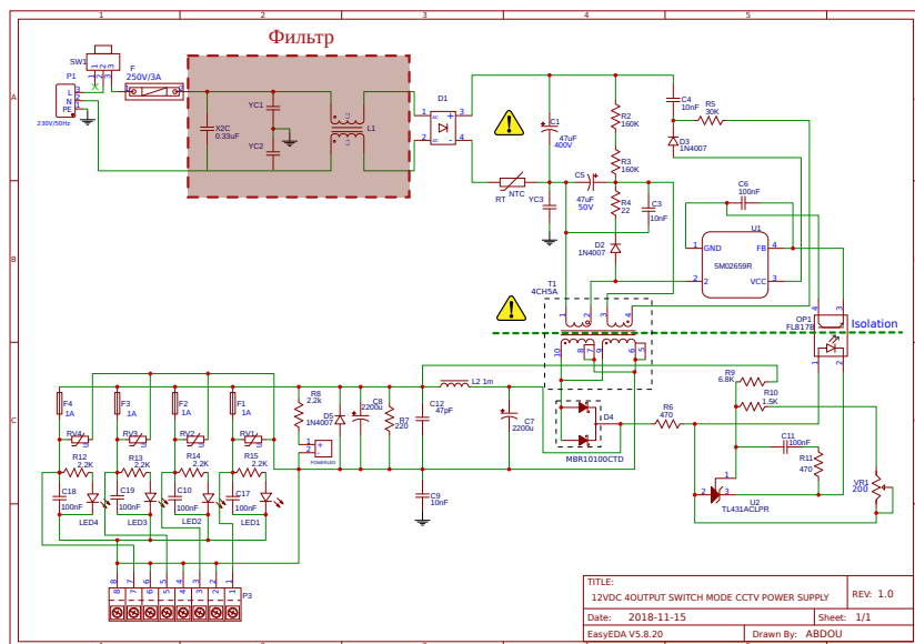
Рисунок 58 Схема импульсного блока питания с сайта oshwlab.com за авторством пользователя abdou. Фильтр я обвёл пунктиром.
