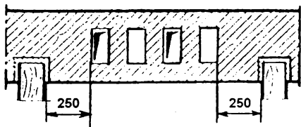
Рис. 116. Изоляция концов балок в печной кладке около каналов
