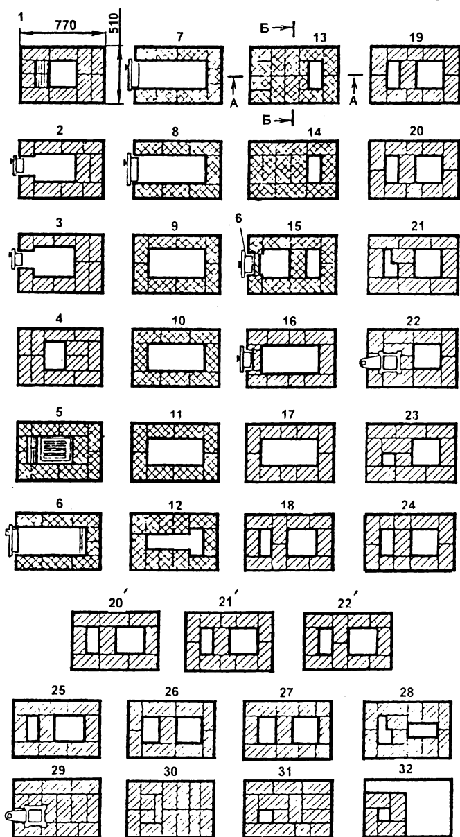
Рис. 92а. Порядовки кладки отопительной печи с теплоотдачей 1760 ккал/ч: 6 - чистка
