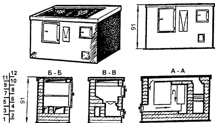
Рис. 73. Кухонная плита с духовкой и водогрейной коробкой производительностью 100 обедов в смену
