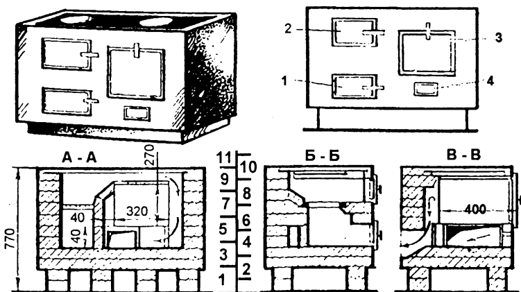
Рис. 69. Кухонная плита на шанцах с духовкой, равномерно обогреваемой со всех сторон: 1 - поддувало; 2 - топливник; 3 - духовка; 4 - чистка
