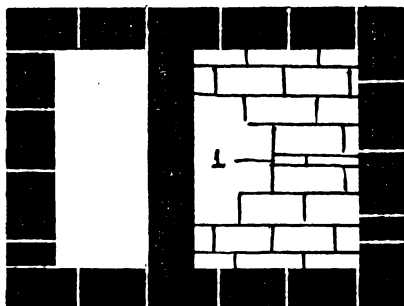
Рис. 40. Кладка свода отдельными захватками: 1 - замковый ряд.
