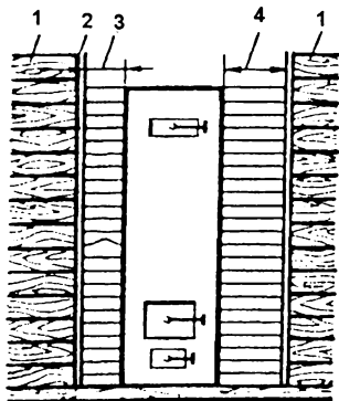
Рис. 114. Отступка между печью и деревянной стеной: 1 - деревянная стена; 2 - кирпичная кладка; 3 - деревянный щит; 4 - два слоя войлока; 5 - вентиляционные решетки; 6 - отступка 13 см
