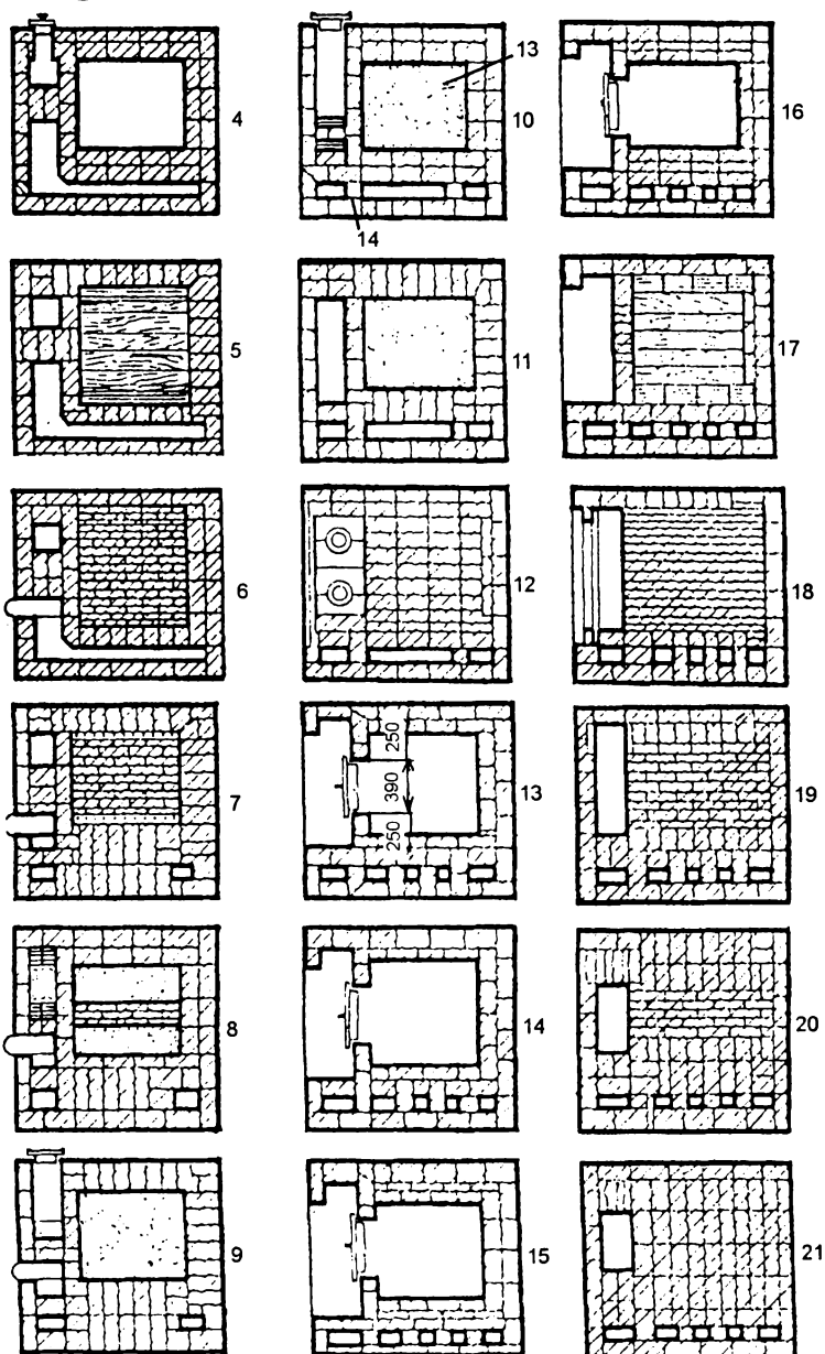
Рис. 89а. Порядовка кладки русской печи с плитой и обогревательным щитком
