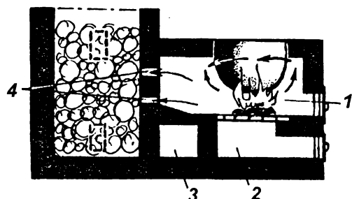
Рис. 62. Печь-каменка с поддувалом:
