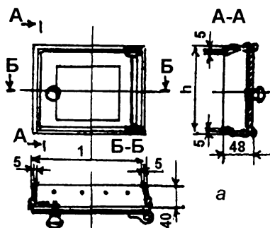
Рис. 5. Дверка обыкновенная
