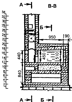
Рис. 87. Русская печь обыкновенная: 1 - гидроизоляция; 2 - мелкий гравий и речной песок, смешанный с битым стеклом
