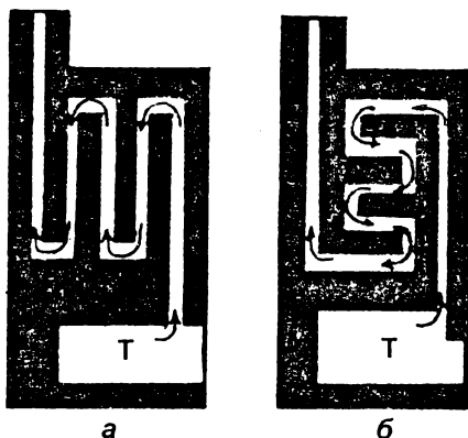
Рис. 49. Многооборотные схемы: а - с вертикальными каналами; б - с горизонтальными каналами; Т - топливник
