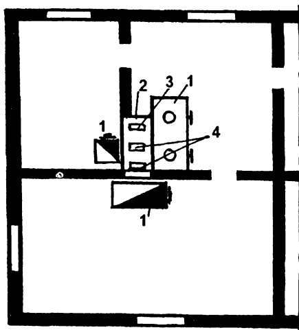
Рис. 24. Подключение печей к коренной трубе:
