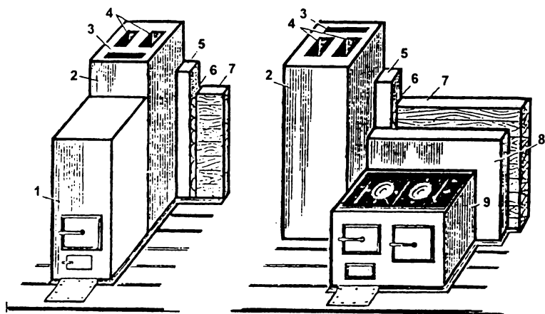
Рис. 99. Коренные трубы с подключенными печами: 1 - печь; 2 - коренная труба; 3 - вентиляционный канал; 4 - дымовые каналы; 5 - разделка; 6 - изоляция из 2-х слоев войлока, вымоченного в глиняном растворе; 7 - стена; 8 - кирпичная стенка; 9 - плита
