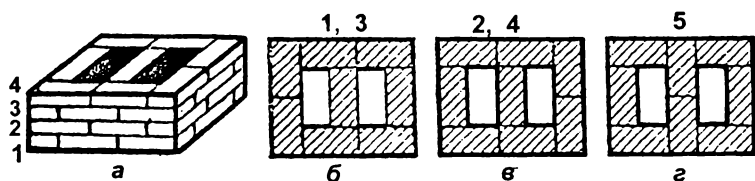
Рис. 104. Кладка трубы при двух спаренных каналах: а - общий вид трубы; б - кладка нечетных рядов; в - кладка четных рядов; г - кладка пятого ряда
