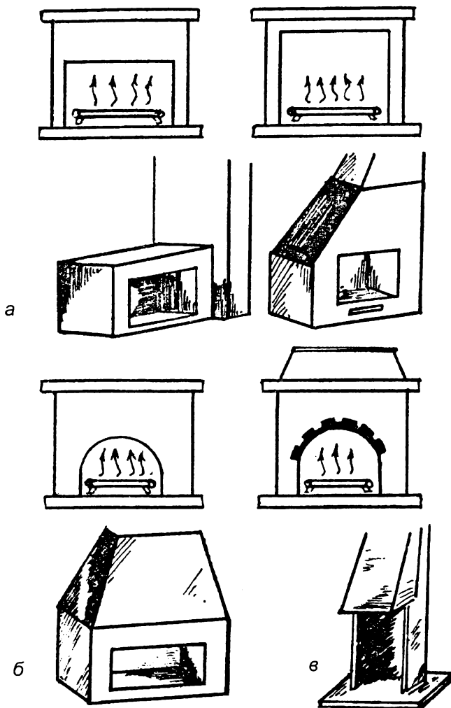
Рис. 55. Разновидности каминов: а - металлические подвесные и напольные; б - металлические и керамические напольные; в - напольные из разных материалов
