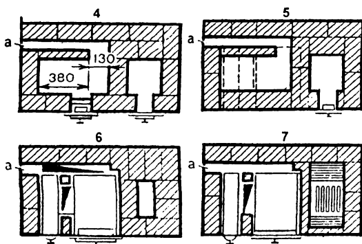
Рис. 71. Варианты отвода дымовых газов с торцевой стороны плиты: а - место присоединения плиты к щитку или дымоходу
