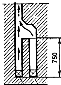
Рис. 100. Присоединение двух печей к одному дымоходу:
