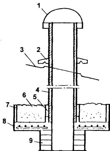
Рис. 111. Асбестоцементная труба:
