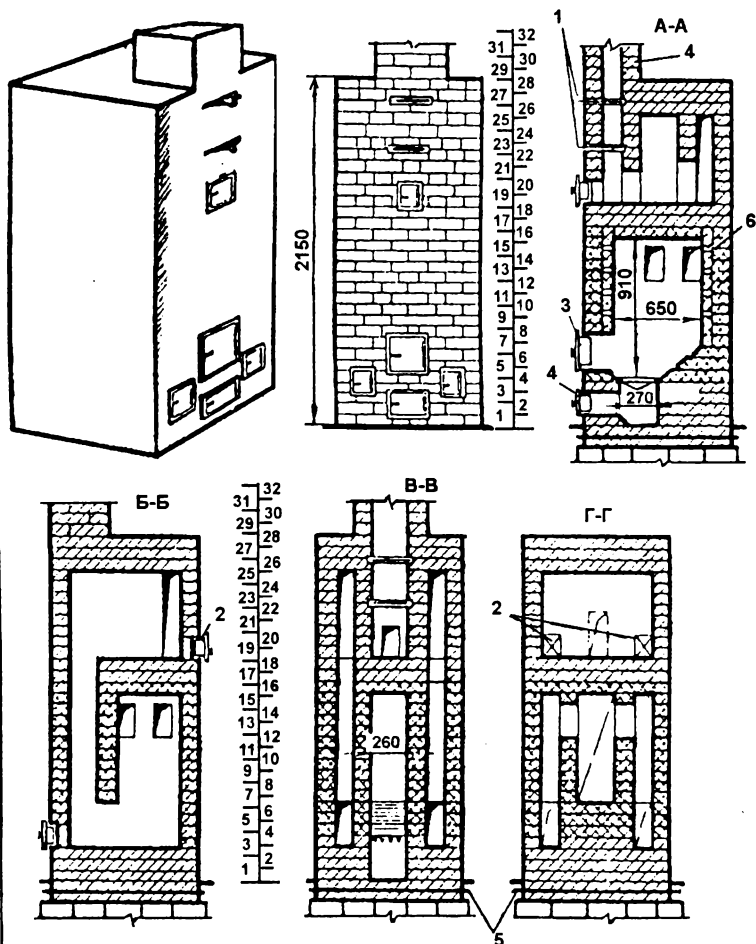
Рис. 96. Отопительная печь, оштукатуренная, с теплоотдачей 3850 ккал/ч: 1 - задвижка; 2 - чистка; 3 - топка; 4 - поддувало; 5 - гидроизоляция; 6 - канал
