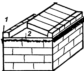
Рис. 32. Укрепление пята треугольного свода путем сжатия угловой или полосовой сталью со стягиванием проволочным жгутом: 1 - тавровая сталь, 2 - проволочный жгут.
