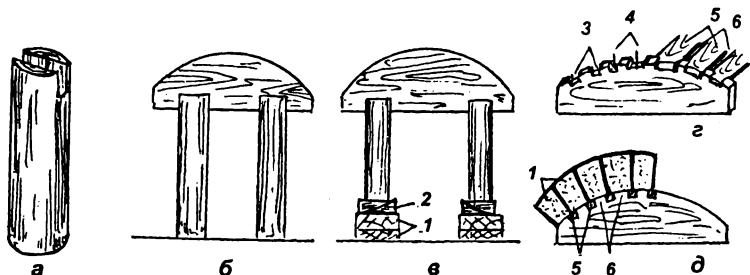
Рис. 38. Устройство разъемной опалубки:
