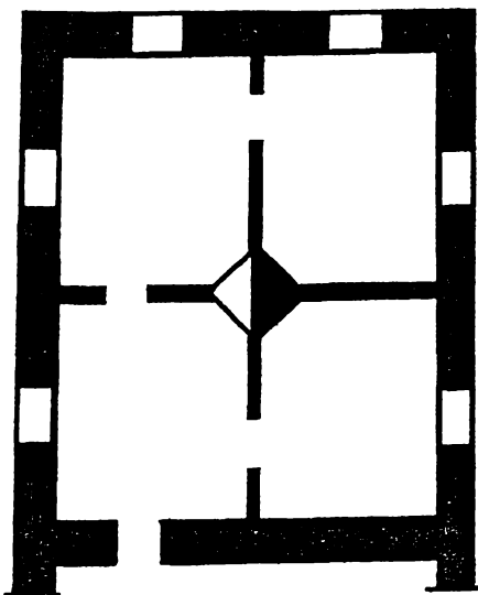
Рис. 23. Установка одной печи для отапливания четырех комнат
