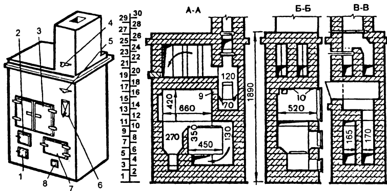
Рис. 81. Отопительно-варочная печь конструкции
