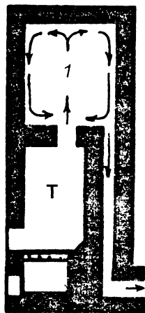
Рис. 50. Бесканальная схема 1 - колпак; Т - топливник
