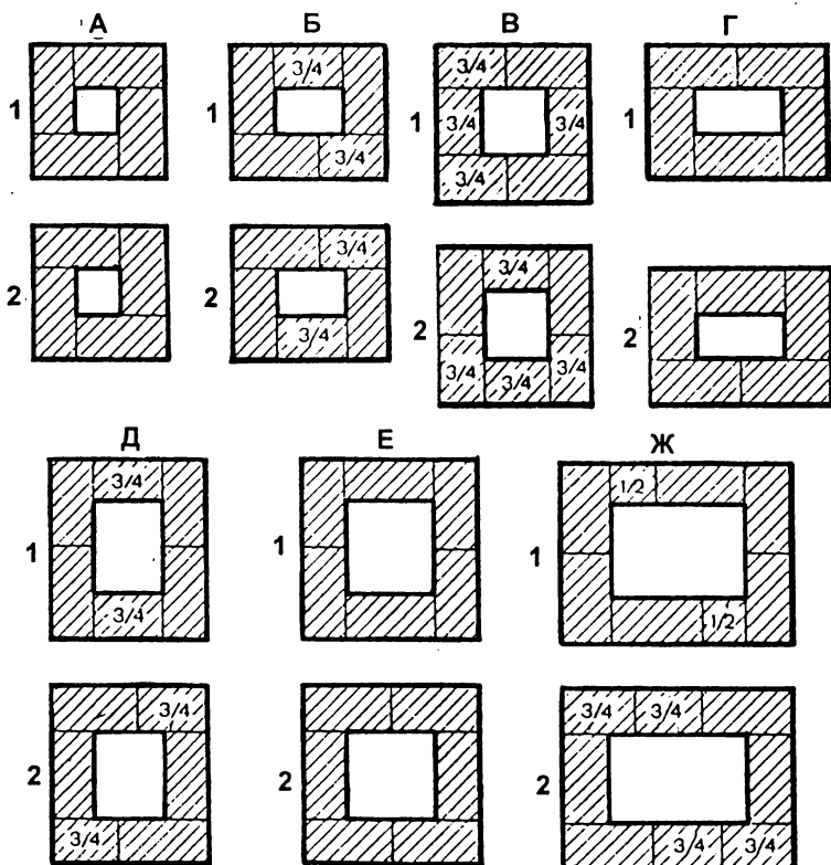
Рис. 103. Размеры дымовых каналов и их кладка: 1 - нечетные ряды; 2 - четные ряды
