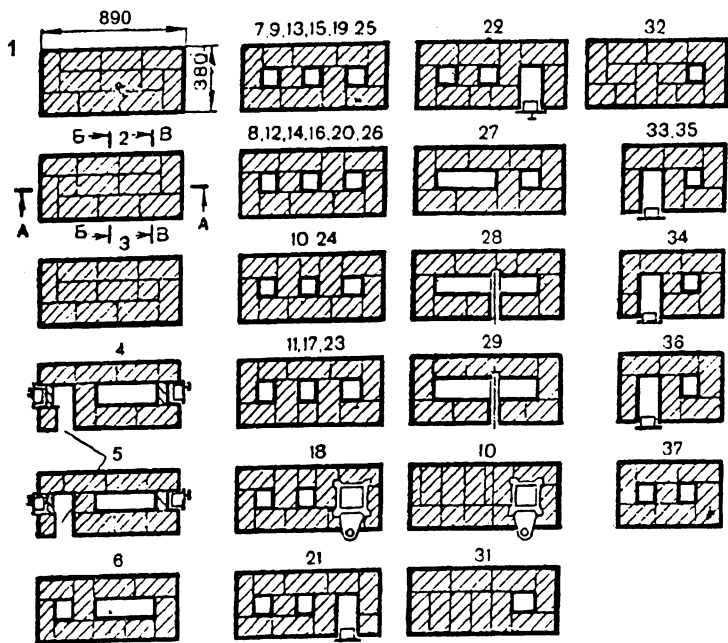
Рис. 77а. Порядовка кладки отопительного толстостенного щитка
