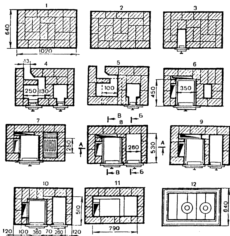
Рис. 68а. Порядовка кладки кухонной печи с духовкой
