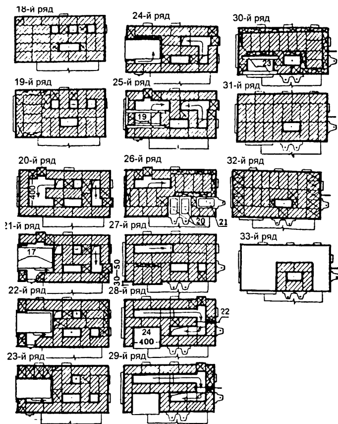
Рис. 656. Порядовка кладки печи-камина с плитой и с духовкой
