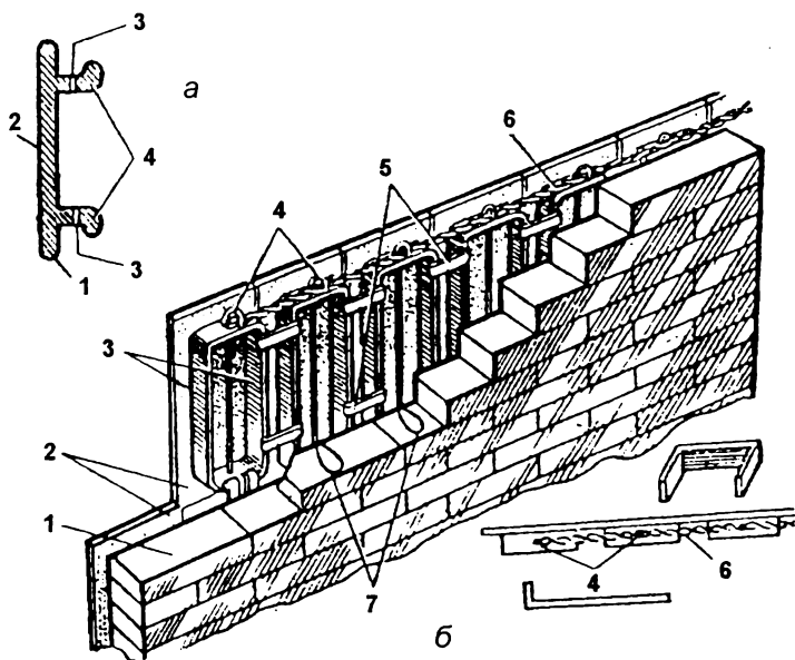
Рис. 112. Облицовка печи изразцами: а - детали изразца: 1 - пластина; 2 - лицо; 3 - отверстия для штырей; 4 - румпа; б - крепление изразцов: 1 - кирпич; 2 - изразцы; 3 - румпа; 4 - штыри; 5 - скобы; 6 - проволоочная вязка; 7 - петля
