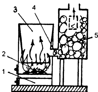
Рис. 63. Печь-каменка из металла:
