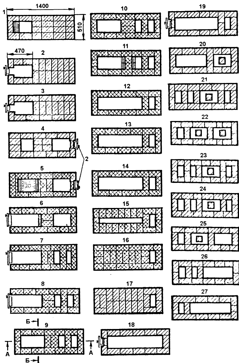
Рис. 94а. Порядовка кладки отопительной печи с теплоотдачей 2400 ккал/ч
