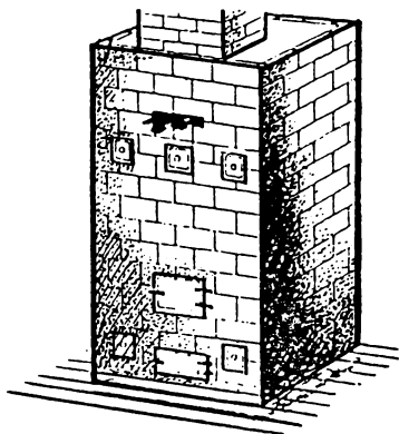
Рис. 98. Отопительная печь изразцовая с теплоотдачей 4150 ккал/ч
