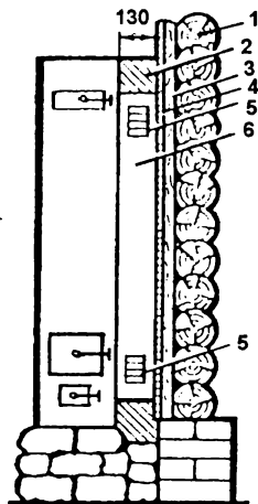
Рис. 114. Отступка между печью и деревянной стеной: 1 - деревянная стена; 2 - кирпичная кладка; 3 - деревянный щит; 4 - два слоя войлока; 5 - вентиляционные решетки; 6 - отступка 13 см
