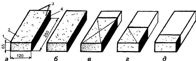
Рис. 19. Кирпич и его части: а - наименование граней кирпича, б - целый, в - трехчетверка, г - половинка, д - четверка, 1 - тычковая грань, 2 - верхняя постель, 3 - ребра (усеки), 4 - ложковая грань
