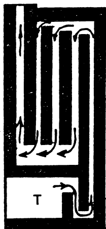
Рис. 51. Схема с преимущественным нижним прогревом: Т - топливник
