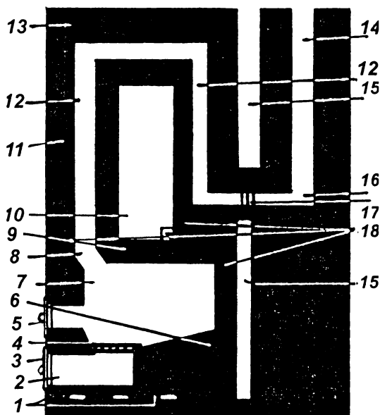
Рис. 41. Схема отопительной печи: 1 - шанцы; 2 - поддувало; 3 - поддувальная дверка; 4 - колосниковая решетка; 5 - топочная дверка; 6 - под; 7 - топочное пространство (топливник); 8 - хайло; 9 - свод топливника; 10 - тепловоздушная камера; 11 - наружная теплоотдающая поверхность; 12 - дымообороты; 13 - перекрыша; 14 - дымоход; 15 - отступка; 16 - патрубок; 17 - задвижка дымовая; 18 - внутренние тепловоспринимающие поверхности.
