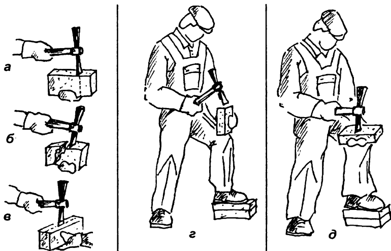
Рис. 26. Колка и теска кирпича: а - правильная колка кирпича поперек, б - неправильная колка поперек, в - колка вдоль, г - рабочее положение при теске, д - рабочее положение при колке
