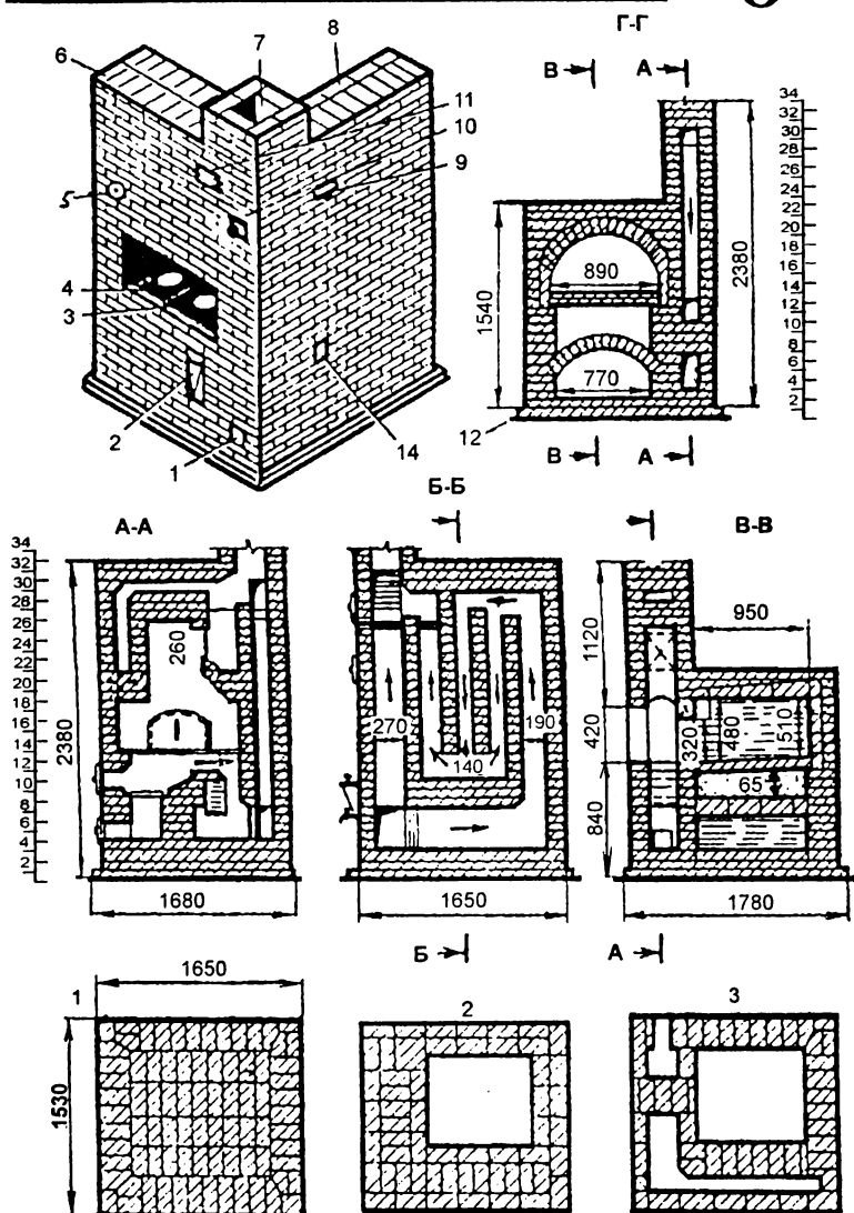
Рис. 81. Русская печь с плитой и обогревательным щитком: 1 - чистка; 2 - водогрейная коробка; 3 - шесток; 4 - чугунная плита; 5 - самоварник; 6 - перекрыша; 7 - труба; 8 - щиток обогревательный; 9, 10 - задвижки; 11 - вьюшка, закрываемая дверкой; 12 - гидроизоляция; 13 - засыпка; 14 - чистка 130x130 мм
