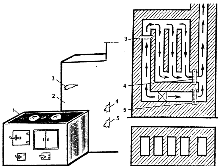
Рис. 76. Разрез щитка с задвижками, расположенными вверху и внизу: 1 - чугунный настил (плита) с двумя конфорками; 2 - щиток; 3 - дымовая задвижка в трубе; 4, 5 - задвижки для регулировки движения газов в летнее и зимнее время
