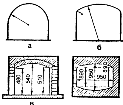
Рис. 86. Форма сводов:
