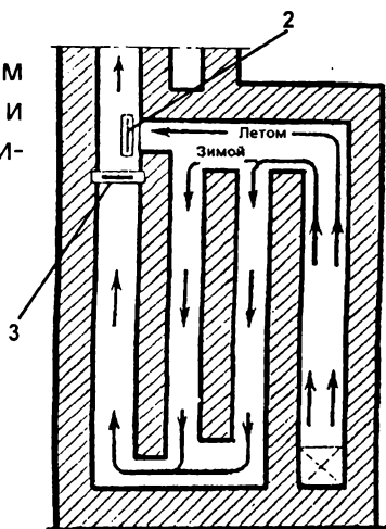
Рис. 75. Отопительный щиток с двумя ходами: зимним и летним
