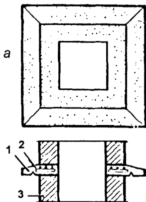
Рис. 110. Изготовление железобетонной выдры: а - выдра в плане; б - положение выдры на трубе; 1 - слезник; 2 - выдра; 3 - печная кладка
