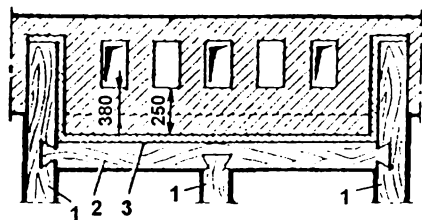
Рис. 117. Устройство ригеля: 1 - балки; 2 - ригель; 3 - изоляция (войлок)
