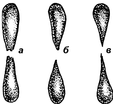
Рис. 2. Проверка на растяжение жгутиков из глиняного раствора: а - тощего, б - нормального, в - жирного
