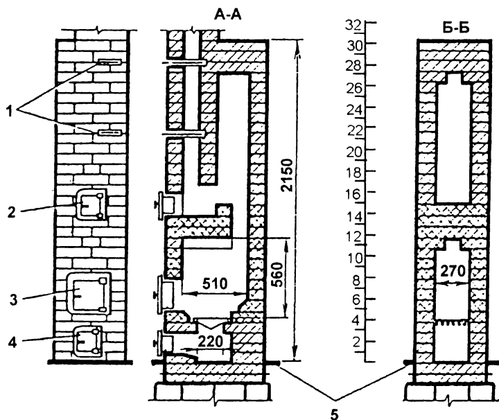
Рис. 92. Оштукатуренная отопительная печь с теплоотдачей 1760 ккал/ч:
