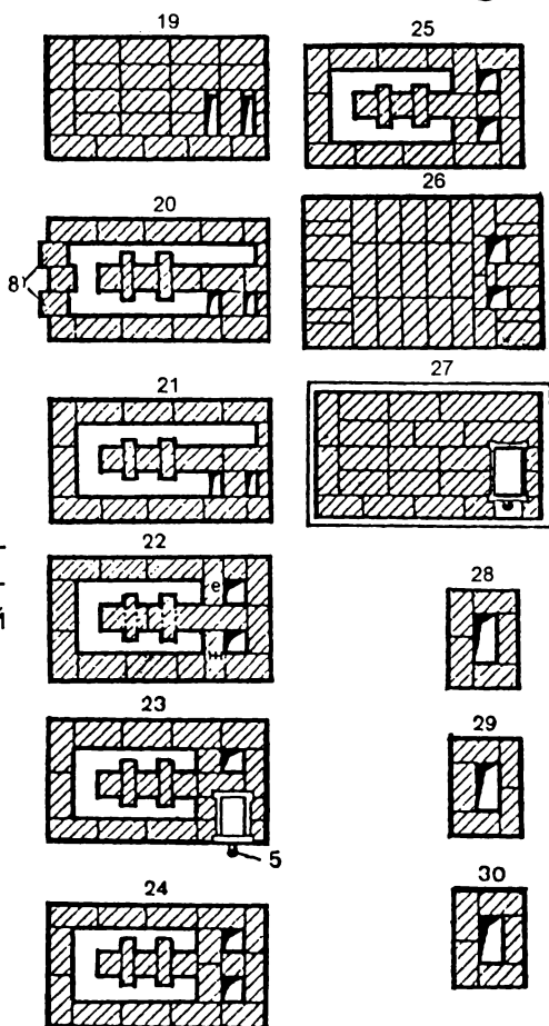
Рис. 81а. Порядовка кладки отопительно-варочной печи конструкции В. А. Потапова (второй вариант)
