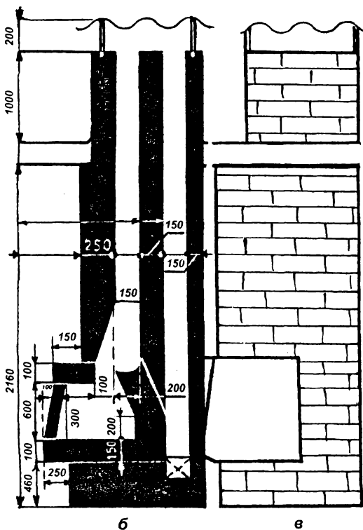
Рис. 57. Камин из кирпича: а - вид спереди; б - разрез; в - вид сбоку
