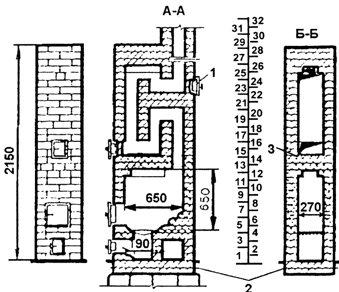
Рис. 93. Отопительная печь. оштукатуренная, с теплоотдачей 1940 ккал/ч.
