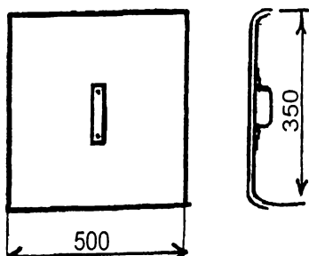
Рис. 12. Заслонка с закругленными краями (по РСТ РСФСР 204-77)
