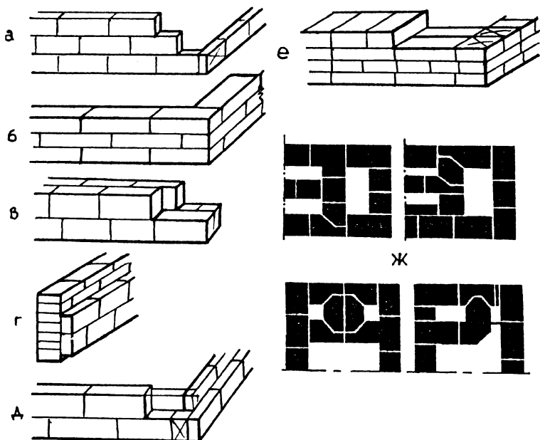
Рис. 21. Печная кладка стенок разной толщины: а - в четверть кирпича, б - в полкирпича (ложком), в - в полкирпича в две четверти, г - в 3/4 кирпича (полкирпича на ребро), д - в полкирпича (2/4 с полным перекрытием швов}, е - в целый кирпич, ж - устройство замков в кладке
