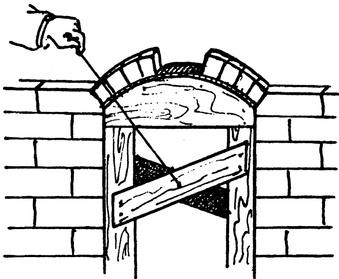
Рис. 39. Проверка правильного расположения швов кладки в арке
