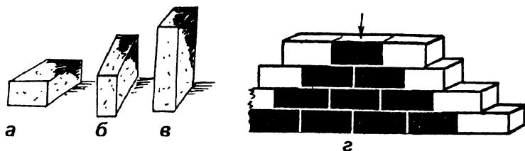
Рис. 20. Укладка кирпича: а - плашня в полкирпича, б - на ребро в четверть кирпича, в - стоя, г - хорошая перевязка швов
