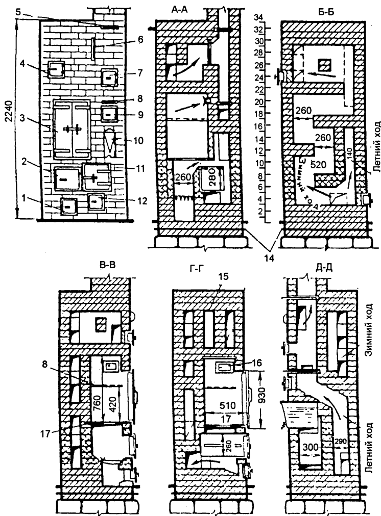
Рис. 83. Отопительно-варочная печь конструкции И. Ф. Волкова: 1 - поддувало; 2 - топка; 3 - варочная камера; 4 - чистка; 5 - дымовая задвижка; 6 - задвижка, открываемая зимой; 7 - самоварник; 8 - задвижка, открываемая летом; 9 - чистка; 10 - водогрейная коробка; 11 - духовка; 12 - чистка; 13 - металлическая сетка в рамке; 14 - гидроизоляция; 15 - замкнутая внутренняя камера; 16 - канал для вентиляции камеры; 17 - чугунные плиты; 18 - вентиляционное отверстие с дверкой
