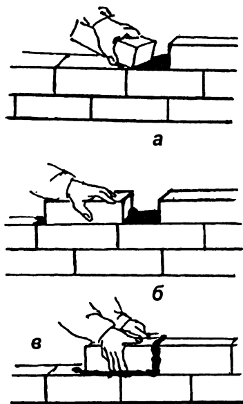
Рис. 28. Укладка кирпича на раствор:
