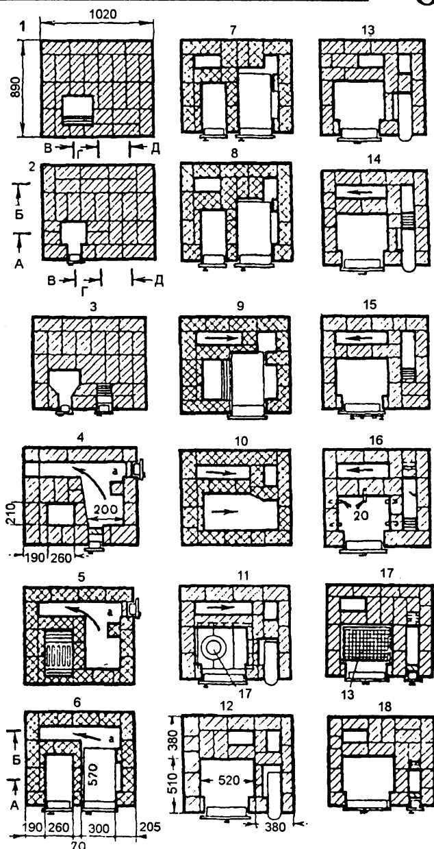
Рис. 83а. Порядовка кладки отопительно-варочной печи конструкции И. Ф. Волкова
