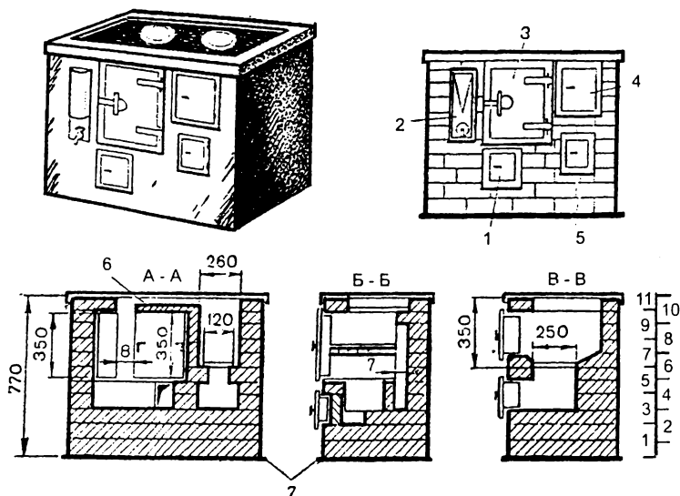
Рис. 70. Кухонная печь упрощенная: 1 - чистка; 2 - водогрейная коробка; 3 - духовка; 4 - топливник; 5 - поддувало; 6 - глиняная смазка толщиной 1-1,5 см; 7 - войлок с кровельной сталью
