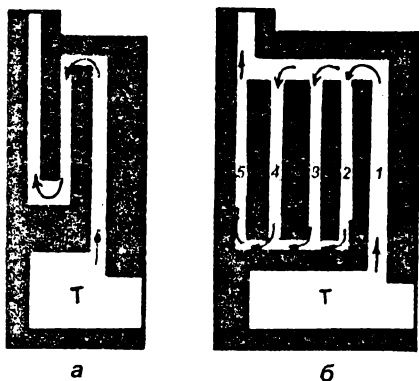
Рис. 48. Малооборотные схемы:
