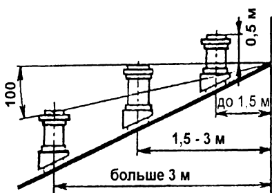
Рис. 102. Расположение труб на крыше
