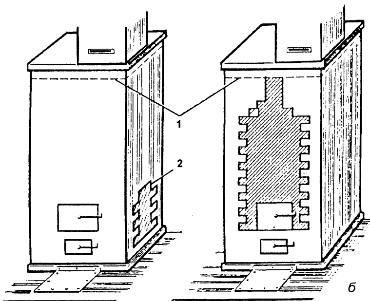
а Рис. 121. Ремонт печей: а - топливника; б - переделка топливника и дымохода: 1 - линия перекрытий печи (перекрыша); 2 - линия перекрытий топливника
