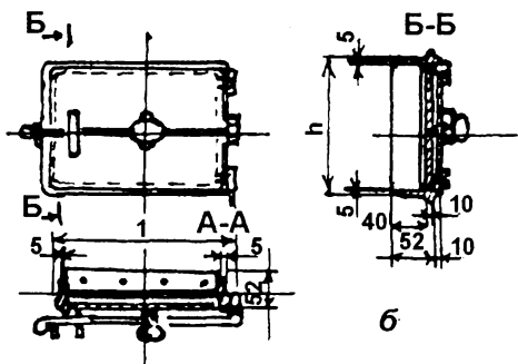
Рис. 8. Дверка герметическая
