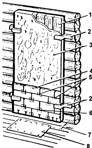
Рис. 113. Изоляция стен от печи:
