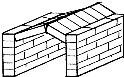
Рис. 31. Перекрытие узкого топливника треугольным сводом
