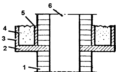
Рис. 109. Изготовление распушки с заполнителем: 1 - печная кладка; 2 - железобетонная плита; 3 - бортовая плита; 4 - заполнитель; 5 - облицовочные плиты вокруг трубы; 6 - дымоход
