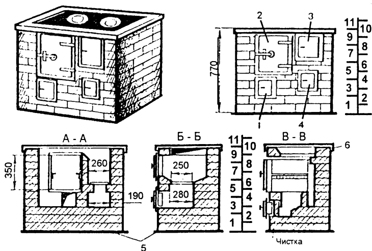
Рис. 68. Кухонная плита с духовкой:
