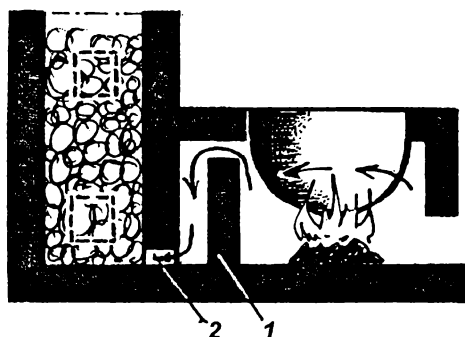
Рис. 61. Улучшенная печь-каменка со стенкой для направления горячих газов:
