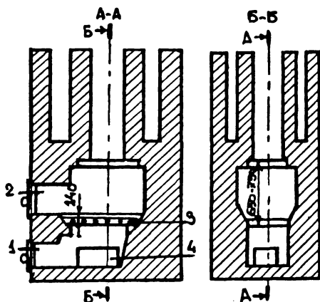
Рис. 44. Топливник для торфа:
