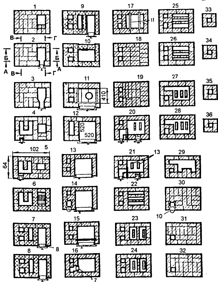
Рис. 82 а. Порядовка кладки обычной отопительно-варочной печи
