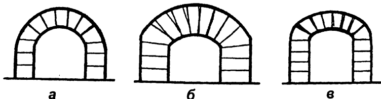
Рис. 35. Форма сводов: а - полуциркульный, б - пологий, в - трехцентровый.
