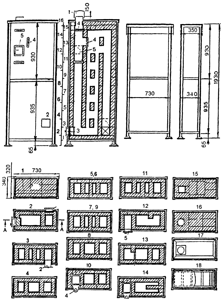
Рис. 78. Отопительный щиток облегченной конструкции в металлическом каркасе, облицованный асбофанерой: 1 - патрубок; 2 - место присоединения плиты к щитку; 3 - чистка; 4 - задвижка; 5 - самоварник
