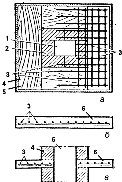
Рис. 108. Изготовление железобетонной выдры: а - опалубка с расположенной арматурой; б - разрез плиты; в - плита в печной кладке; 1 - дымоход; 2 - печная кладка; 3 - арматура; 4 - бортики; 5 - опалубка; 6 - плита
