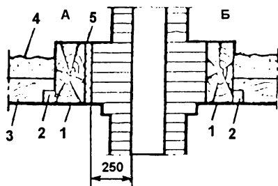
Рис. 118. Разделка распушки в чердачном перекрытии:
