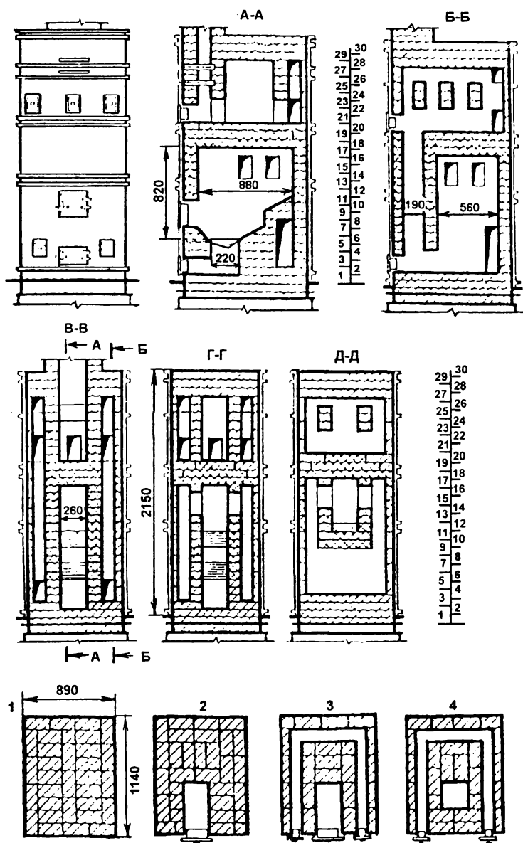
Рис. 97а. Отопительная печь в металлическом футляре с теплоотдачей 3920 ккал/ч и порядовка кладки
