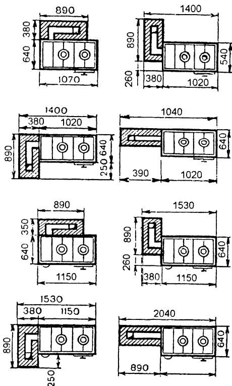
Рис. 72. Схемы присоединения плиты к отопительным щиткам
