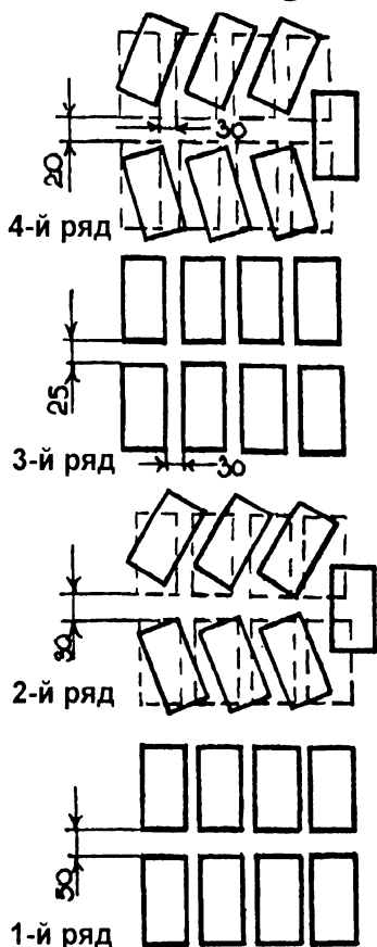
Рис. 4. Схема укладки кирпича для сушки
