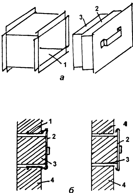
Рис. 10. Чистки-коробочки: а - общий вид, б - коробочка, вставленная в кладку, 1, 1 - рамка, 2 - коробочка, 3 - кирпич, 4 - печная кладка
