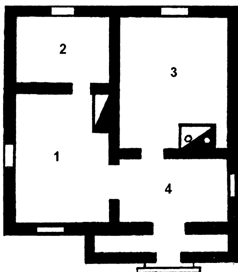
Рис. 25. Установка печей в комнатах дома и их подбор на теплоотдачу:
