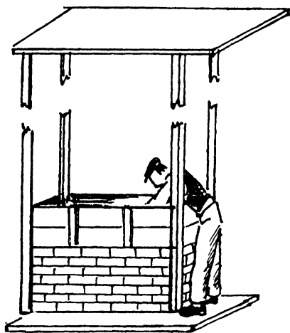
Рис. 18. Кладка печи в подвижной опалубке
