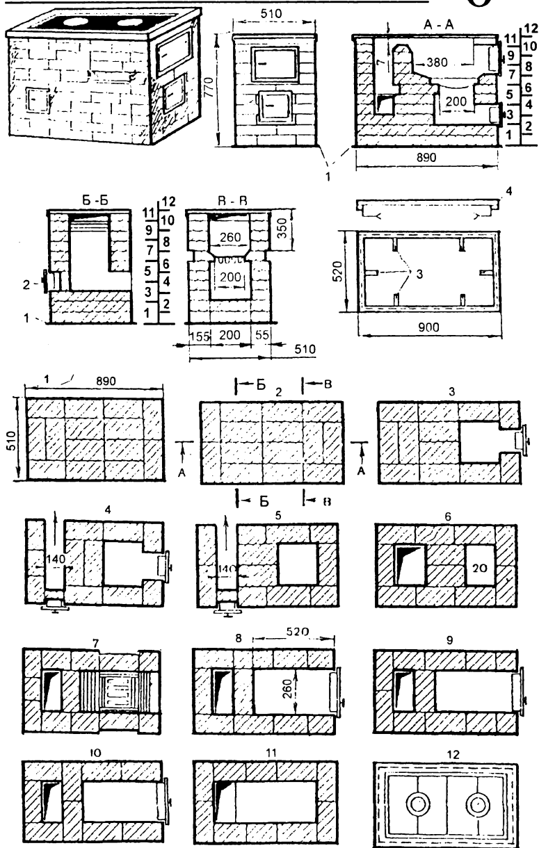
Рис. 67. Кухонная печь упрощенная: 1 - два слоя войлока; 2 - чистка; 3 - кляммеры; 4 - угловая сталь 30x30x4 мм с укрепленными кляммерами из стальной ленты.
