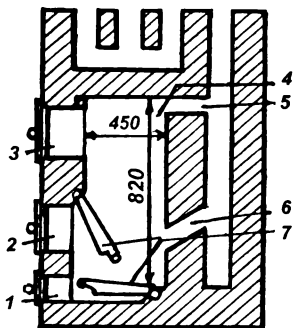
Рис. 45. Топливник для торфа повышенной влажности:
