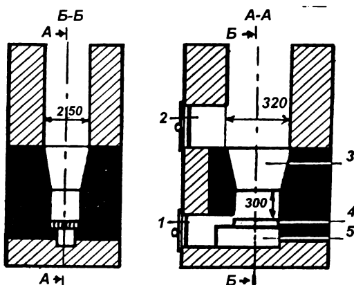
Рис. 46. Топливник для каменного угля: 1 - поддувало; 2 - топливник; 3 - шахта; 4 - колосниковая решетка; 5 - металлический ящик для сбора золы.
