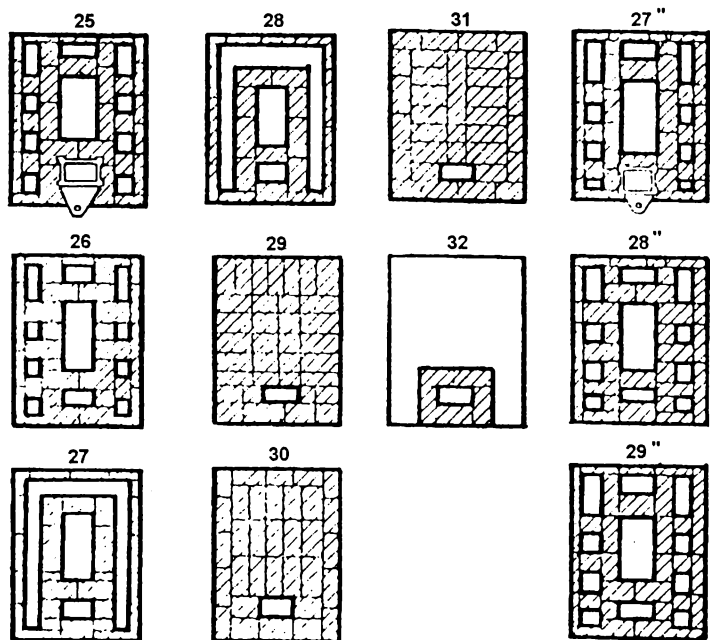
Рис. 976. Порядовка кладки отопительной печи в металлическом футляре с теплоотдачей 2400 ккал/ч (продолжение, начало см. стр. 255-256)
