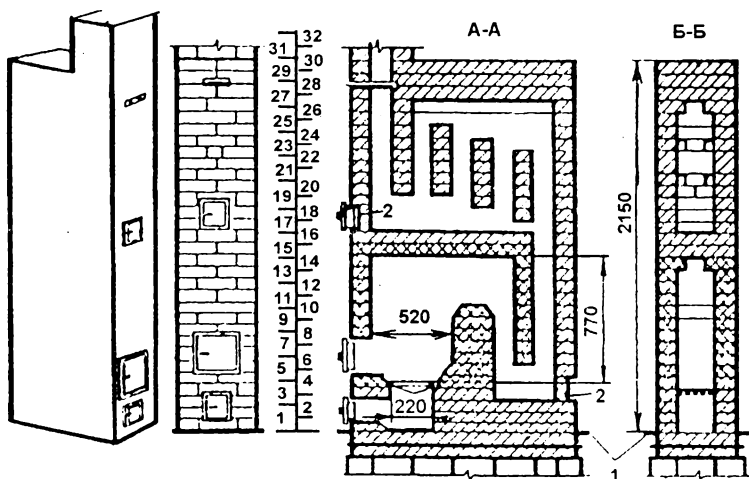
Рис. 94. Отопительная печь, оштукатуренная, с теплоотдачей 2400 ккал/ч:
