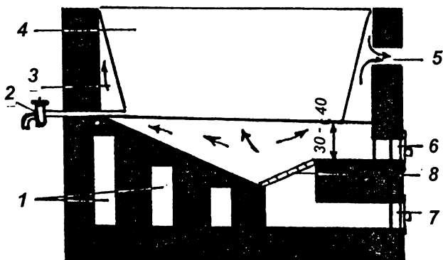
Рис. 58. Банная печь с котлом для нагревания воды: 1 - канал для выхода тепла; 2 - кран; 3 - пазуха для горячих газов; 4 - котел; 5 - канал для отвода газов в трубу; 6 - топочная дверка; 7 - поддувальная дверка; 8 - колосниковая решетка
