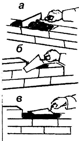
Рис. 29. Работа кельмой:
