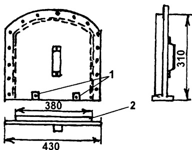
Рис. 13. Заслонка, применяемая в старых печах,
