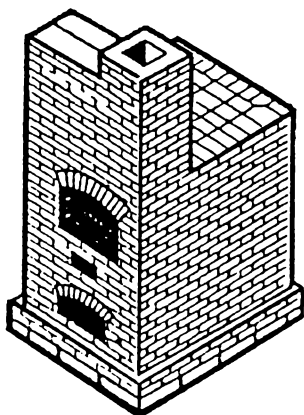
Рис. 87. Русская печь обыкновенная: 1 - гидроизоляция; 2 - мелкий гравий и речной песок, смешанный с битым стеклом
