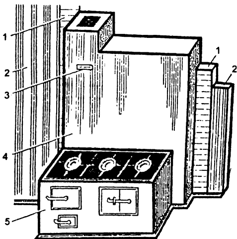
Рис. 74. Кухонная плита с постоянно нагреваемым отопительным щитком: 1 - кирпичная разделка; 2 - перегородки (стенки); 3 - дымовая задвижка; 4 - щиток; 5 - плита
