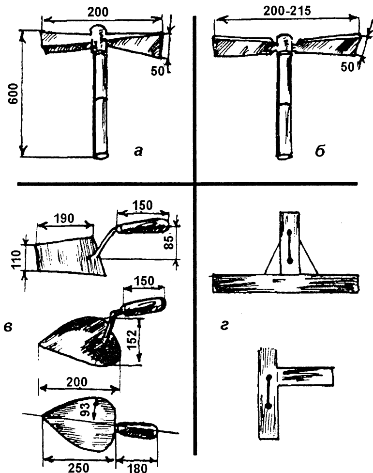
Рис. 14. Инструменты для печных работ: а - печной молоток, б - кирочка, в - кельма, г - ватерпас
