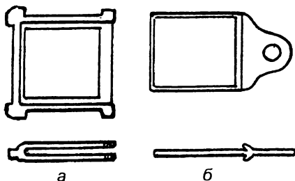
Рис. 6. Задвижка печная: а - рамка, б - движок
