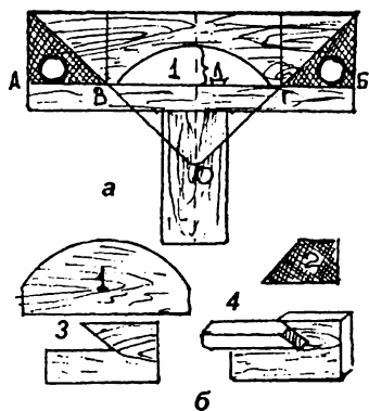
Рис. 36. Построение кружала для свода и шаблона для пят: а - построение кружала, б - кружало и шаблоны, 1 - кружало, 2 - шаблон пяты, 3 - шаблон для тески пят, 4 - проверка отесанного кирпича
