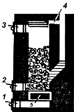
Рис. 47. Топливник шахтный для каменного угля:
