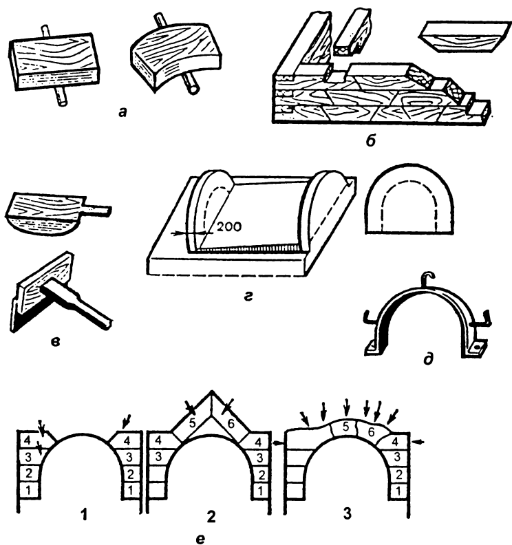
Рис. 91. Приспособления и порядок устройства русской глинобитной печи;
