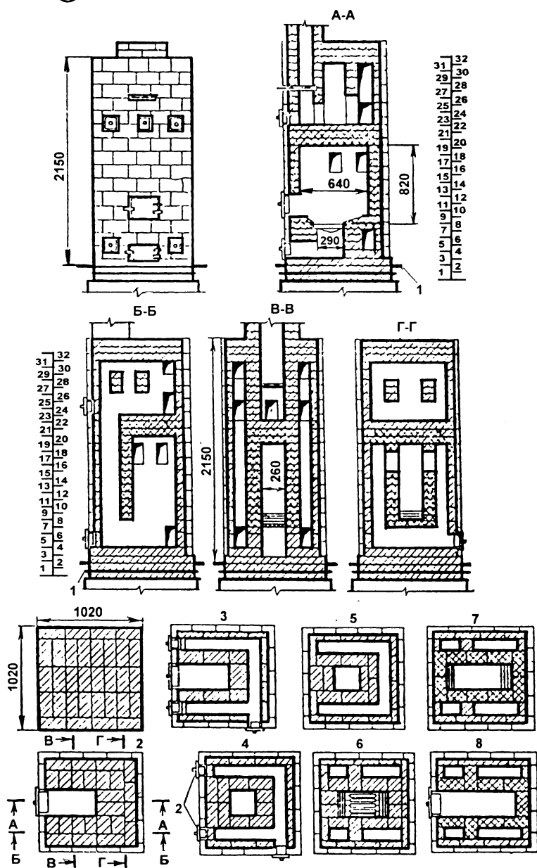
Рис. 98а. Отопительная печь изразцовая с теплоотдачей 4150 ккал/ч: 1 - гидроизоляция; 2 - чистка
