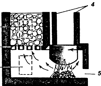
Рис. 59. Банная печь-каменка: 1, 3 - дверки; 2 - чугунные брусья; 4 - проволока или тросик; 5 - топливник
