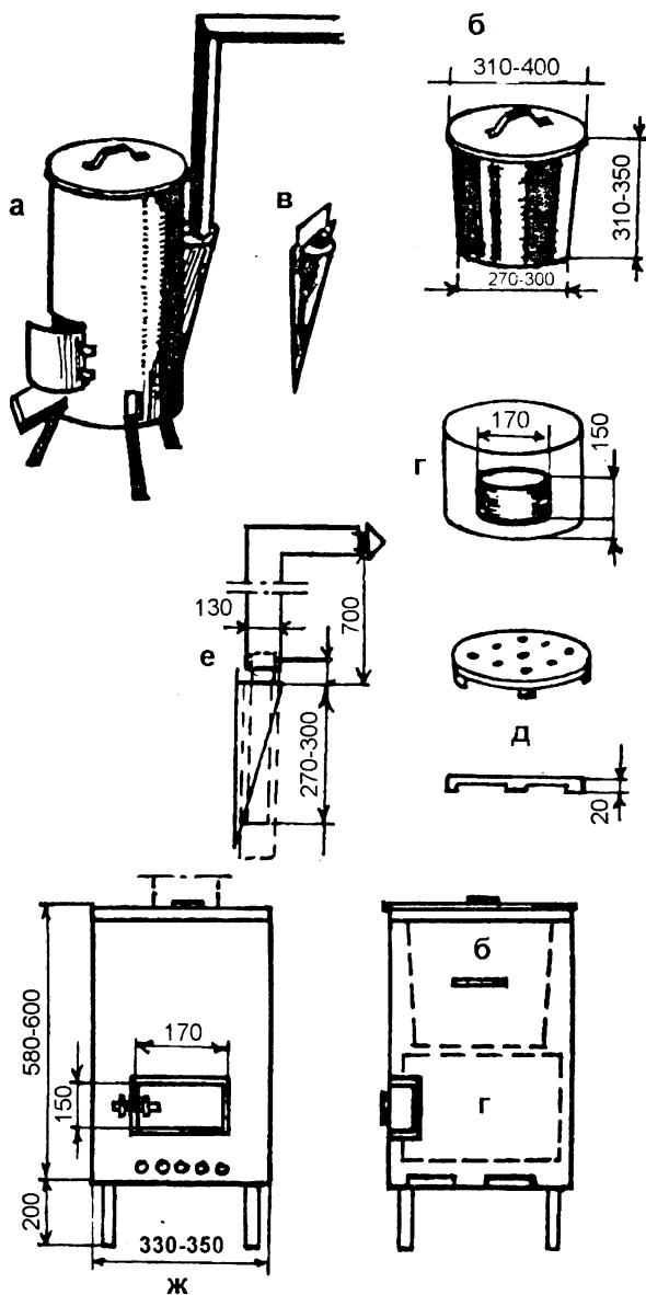
Рис. 64. Печь-прачка:
