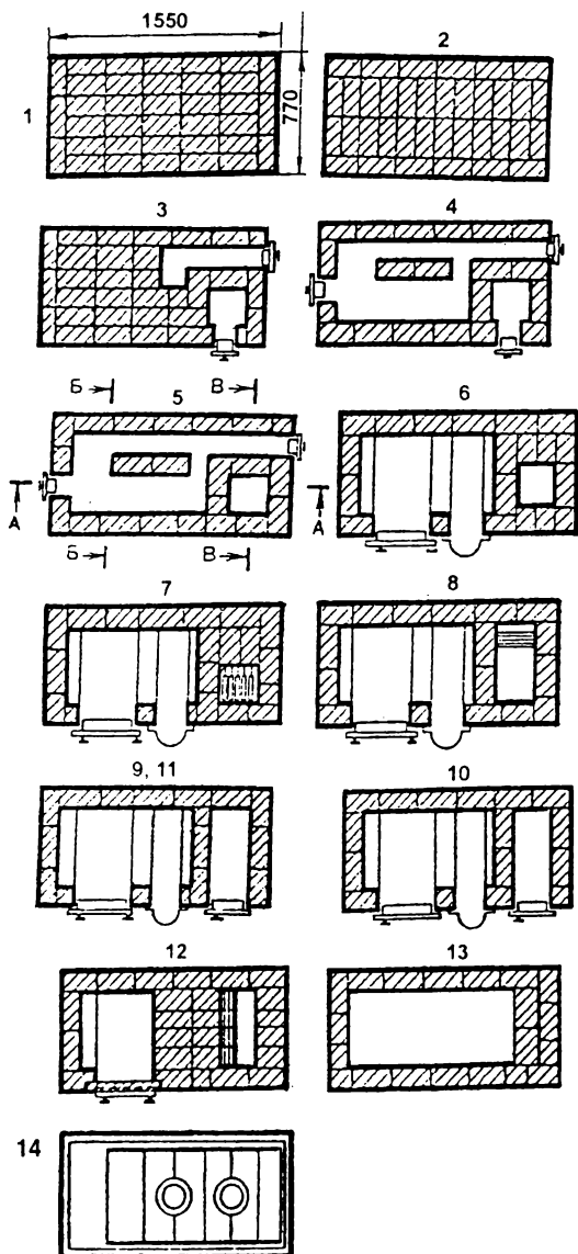
Рис. 73а. Порядовка кладки кухонной плиты с духовкой и водогрейной коробкой производительностью 100 обедов в смену
