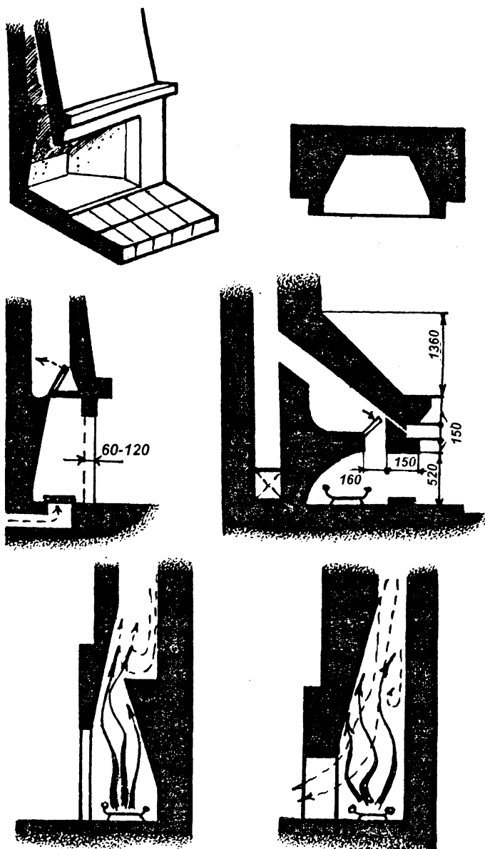
Рис. 53. Разрезы каминов и форма газовых порогов
