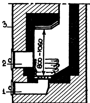
Рис. 42. Топливник для дров:
