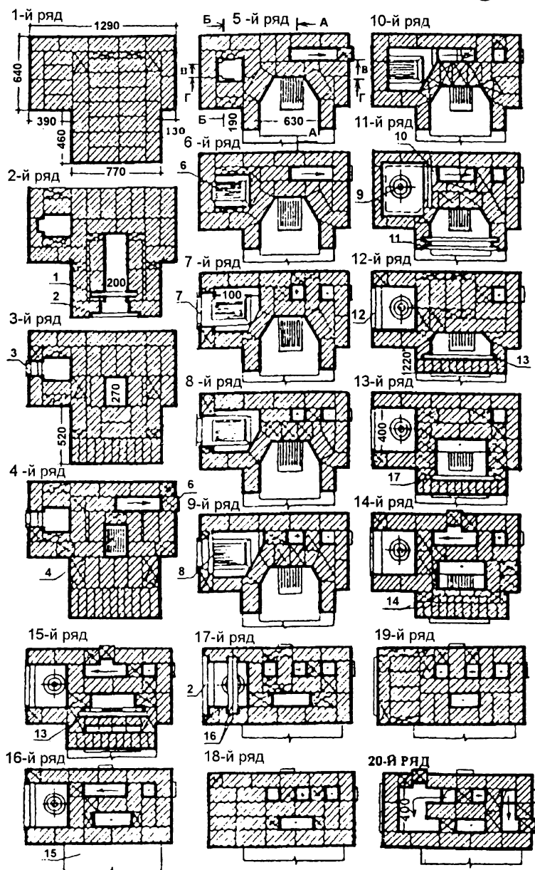
Рис. 656. Порядовка кладки печи-камина с плитой и с духовкой
