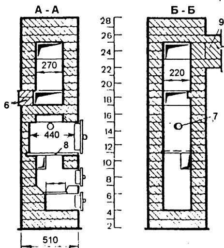
Рис. 80. Отопительно-варочная печь конструкции В. А. Потапова (первый вариант):
