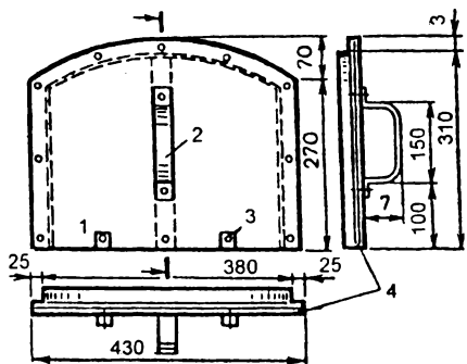
Рис. 88. Заслонка:
