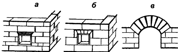
Рис. 34. Перекрытие проемов печей и топливников над топочными дверками:
