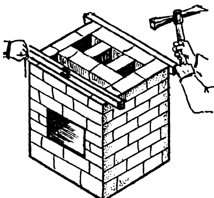
Рис. 17. Проверка выполненной печной кладки
