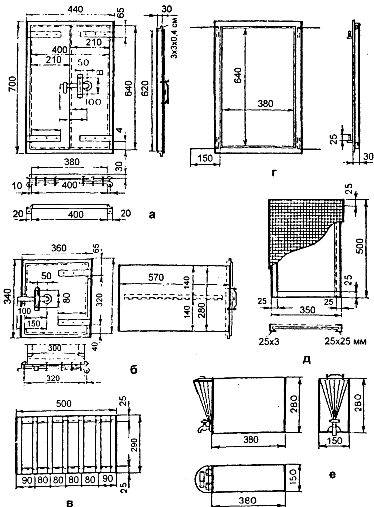
Рис. 84. Изготовление дверей, решеток, водогрейной коробки для отопительно-варочной печи:
