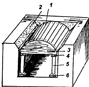
Рис. 37. Опалубка для кладки сводов:
