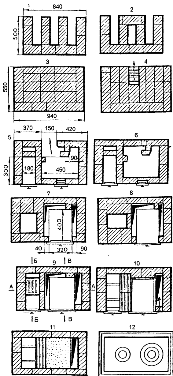
Рис. 69 а. Порядовка кладки кухонной плиты на шанцах
