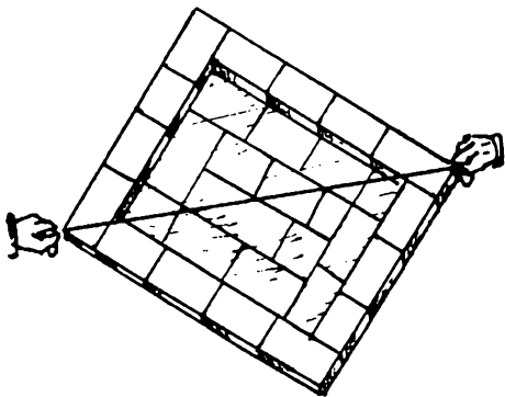
Рис. 16. Проверка закладки первого ряда кладки печи
