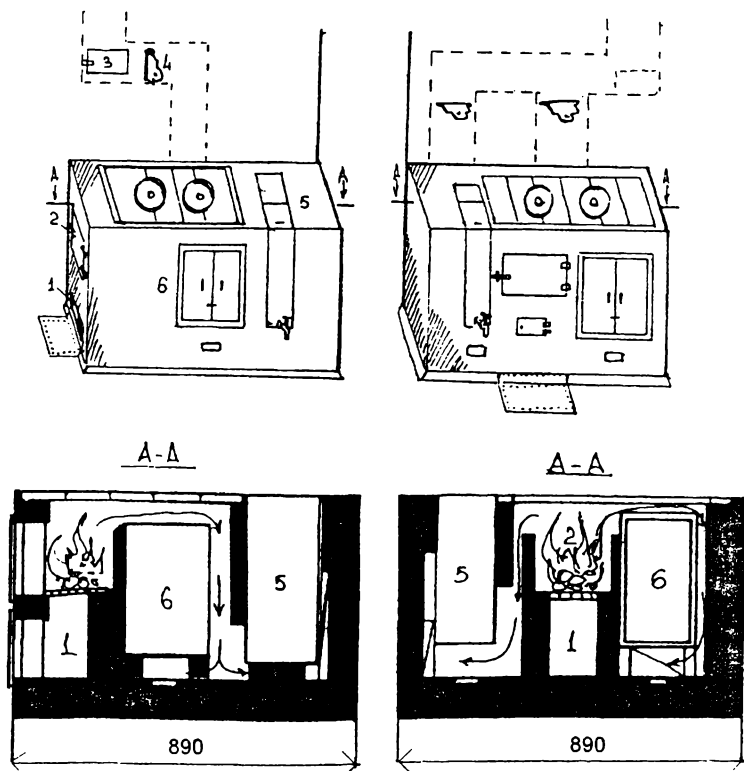
Рис. 66. Кухонная печь:
