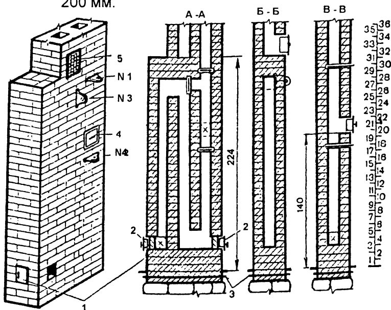
Рис. 77. Отопительный щиток толстостенный:
