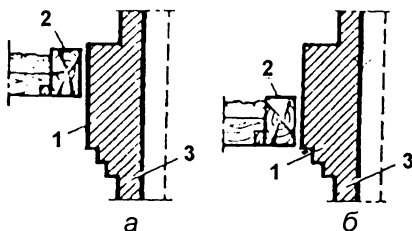
Рис. 120. Расположение распушки с учетом осадки перекрытия: а - до осадки; б - после осадки; 1 - распушка; 2 - перекрытие; 3 - стояк трубы
