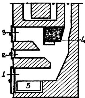
Рис. 43. Топливник для сланцев:
