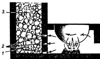
Рис. 60. Улучшенная печь-каменка: 1, 3 - дверки; 2 - отверстие в стене топливника
