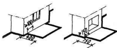
Рис. 71. Установка предтопочного металлического листа
