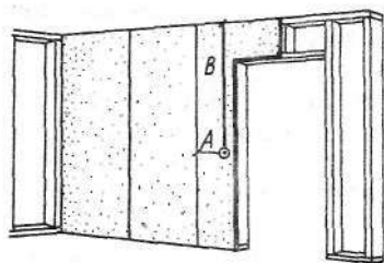
Рис. 151. Разметка положения отверстия для электрической розетки
