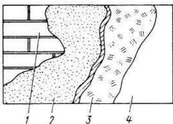
Рис. 205. Слои штукатурки
