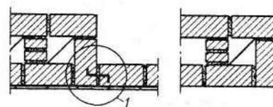
Рис. 193. Соединение простенка трубы и пожарной стены (лицевая кладка может быть выполнена с обеих сторон) 1 — через каждые 8 — 10 швов
