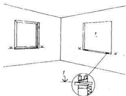
Рис. 165. Укрепление оконных коробок с помощью клиньев 1 — пробки оконного поема
