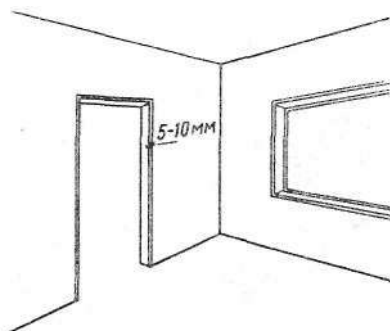
Рис. 230. Границы окраски откосов оконных и дверных проемов
