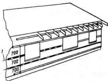
Рис. 134. Расположение продольных брусев или досок с гвоздевыми креплениями под облицовку вертикальными листами или плитами 1 — разметочная линия, нанесенная с помощью мелованного шнура
