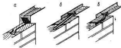
Рис. 199. Способы крепления печной дверцы а — лапкой, поставляемой в комплекте с дверцей; б — проволоочной петлей; в — пластиной из жести
