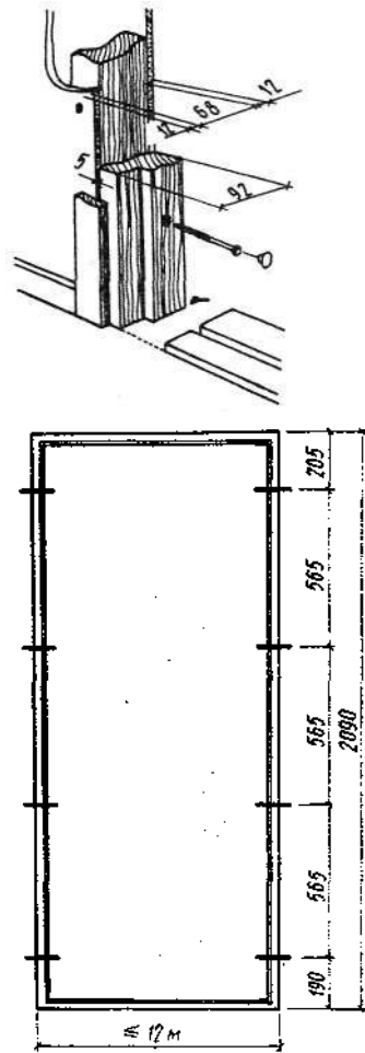
Рис. 169. Места и способ крепления дверных коробок
