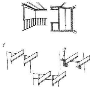
Рис. 146. Установка пароизоляционного слоя на внутренней стороне наружных стен и способ уплотнения проходов балок перекрытия 1 — продление пароизоляции на стыке перекрытия и стены; 2 — клейкая лента
