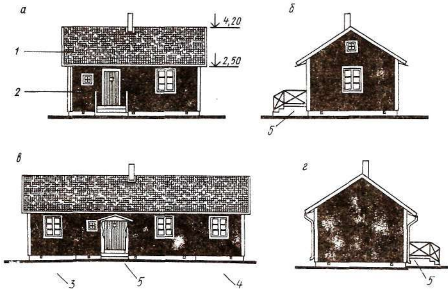
Рис. 17. Проекция фасадов дома
