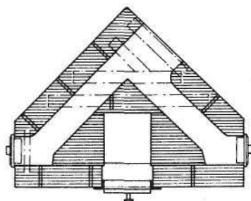
Рис. 201. Выполнение каналов дымоходов с помощью полосовой стали
