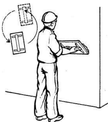
Рис. 207. Применение полутерки при доводке поверхности
