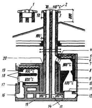
Рис. 70. Пример объединенной шахты дымохода для двух рядом расположенных печи и камина
