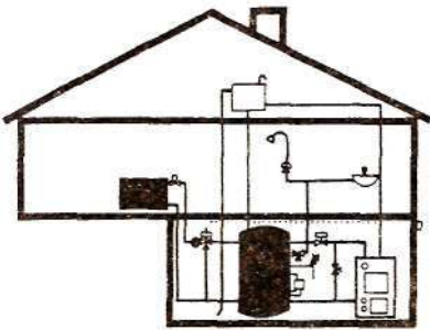
Рис. 61. Система водяного отопления и горячего водоснабжения
