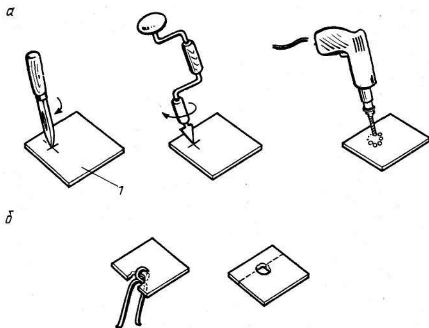
Рис. 222. Способы проделывания отверстий в плитке
