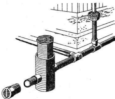
Рис. 236. Размещение дренажных канав, если сток с крыши направляют в дренажные канавы
