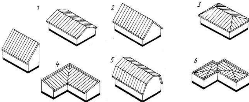
Рис. 37. Типы крыш
