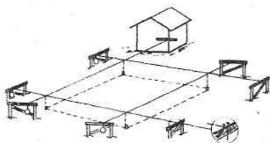
Рис. 90. Расположение на строительной площадке опор (обносков) для вешек и крепления разметочных шнуров
