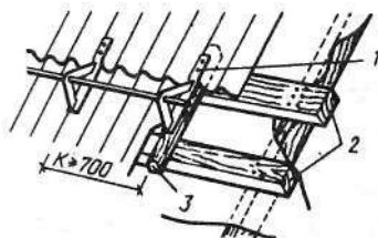
Рис. 128. Крепление конструкций снегозадержателя 1 — оцинкованный гвоздь или шуруп; 2 — дополнительная слега; 3 — опорная рейка
