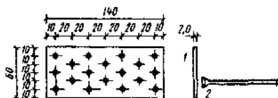
Рис. 50. Прямые пластины для гвоздевых сое- динений деревянных элементов 1 — оцинкованная сталь; 2 — ребристые гвозди
