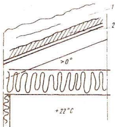
Рис. 260. Образование льда на крыше либо из-за слабой изоляции, либо из-за плохой вентиляции
