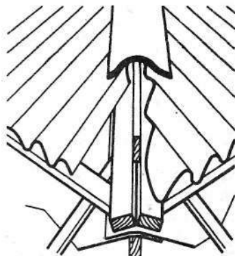
Рис. 126. Выполнение покрытия ребра вальмовой кровли
