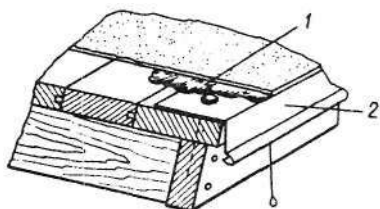
Рис. 117. Использование жести и покрытий пластиком на толевых кровлях 1 — слой битумной мастики; 2 — фасонный элемент из тонкого листа кровельной жести на карнизном свесе
