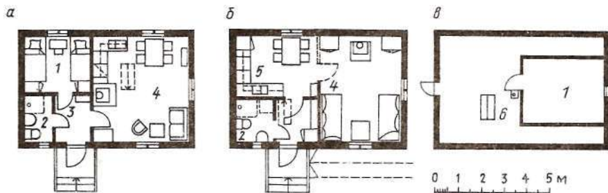
Рис. 15. План этажа
