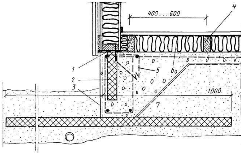
Рис. 53. Узел соединения наружной стеновой панели с монолитной плитой фундамента, усиленной боковой балкой
