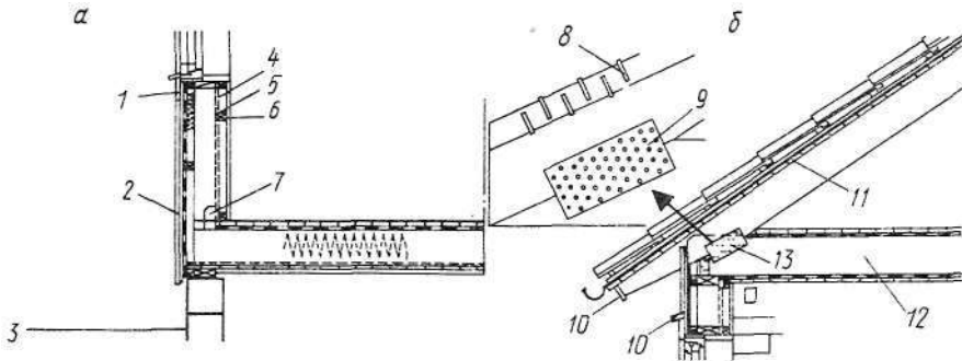
Рис. 18. Примеры чертежей узлов
