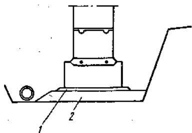
Рис. 177. Установка блоков основания на прочном грунте 1 — песок или раствор; 2 — уплотненный гравий
