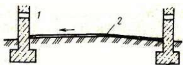
Рис. 259. Правильно запроектированная и закрытая пластиком поверхность грунта
