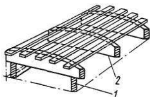
Рис. 200. Опалубка для кладки арочных сводов печей
