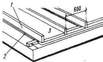
Рис. 55. Выполнение теплоизоляционного слоя в конструкции междуэтажного или цокольного перекрытия
