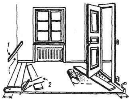
Рис. 158. Раскладка досок настила пола 1 — плинтус; 2 — подсчитать требуемое количество досок
