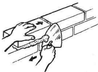
Рис. 184. Положение мастерка при сбросе лишнего раствора
