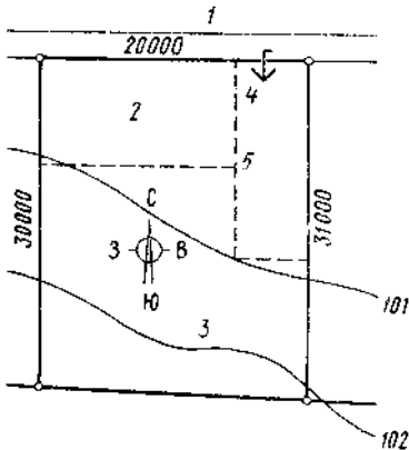
Рис. 5. Пример расположения зон на земельном участке
