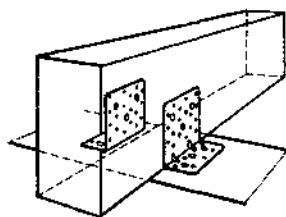
Рис. 49. Использование угловых крепежных элементов при установке балок или стропил крыши Гвозди расположены наиболее выгодно с точ- ки зрения нагрузки
