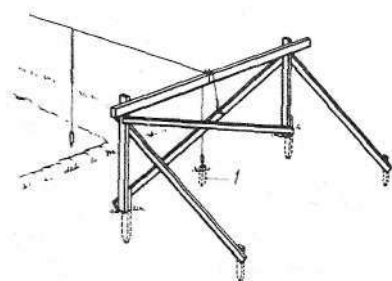
Рис. 91. Конструкция опор (обносков) для установки вешек и крепления шнуров 1 — причалка
