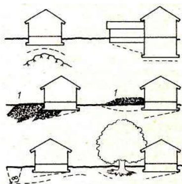
Рис. 263. Провал фундамента вызывается вследствие различного состава грунта в основании здания, различиями в нагрузках, недостаточно тщательно уплотненной засыпкой, изменением уровня грунтовых вод 1 — насыпной грунт
