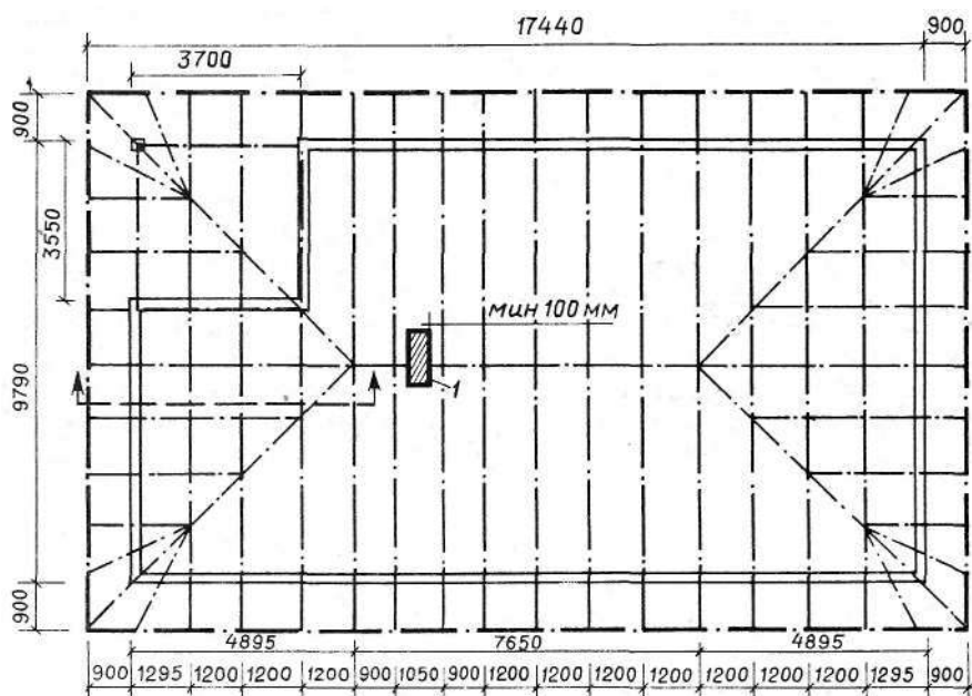
Рис. 40. План расположения ферм и стропил при устройстве четырехскатной вальмовой крыши 1 — дымовая труба
