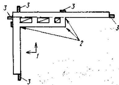
Рис. 192. Кладка дымоходов и труб 1 — лицевая кладка; 2 — углы, выложенные с помощью отвеса; 3 — порядовки
