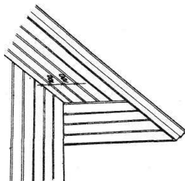
Рис. 141. Обшивка карнизного свеса досками. Наиболее узкая облицовочная доска помещена около стены
