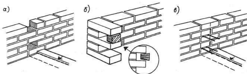
Рис. 190. Виды соединений каменной кладки
