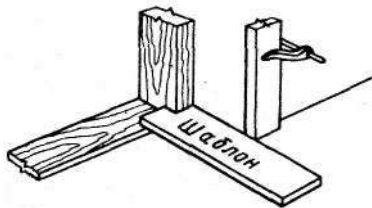
Рис. 212. Применение шаблона при штукатурке откосов
