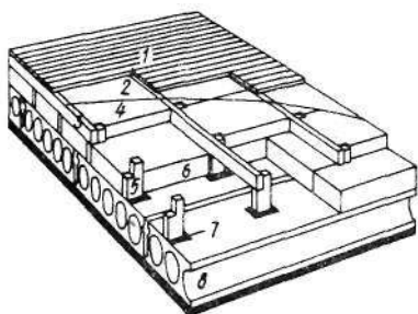
Рис. 54. Конструкция основания с использованием многоспустых плит
