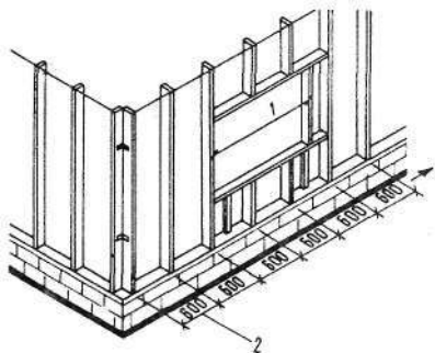
Рис. 101. Установка вертикальных брусков каркаса при бесшовной облицовке. В местах стыков облицовки надо поставить дополнительные вертикальные брусочки
