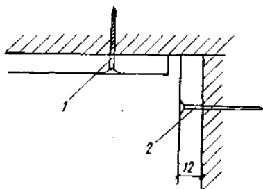
Рис. 148. Размеры гвоздей и шурупов при креплении плит облицовки 1 — шуруп на потолке 30 — 35 мм; 2 — гвоздь для стены 90 x 1,7
