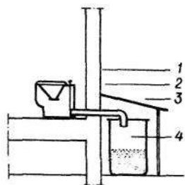
Рис. 240. Химический туалет
