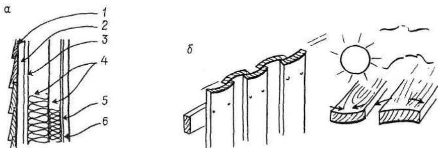
Рис. 29. Внешняя облицовка стен подвергается наибольшему климатическому воздействию а — конструкция наружной стены; б — конструкция обшивки; 1 — наружная облицовка; 2 — деревянная рейка для крепления; 3 — пленка для защиты от промерзания; 4 — минеральная вата; 5 — пароизоляционный слой; 6 — внутренняя обшивка
