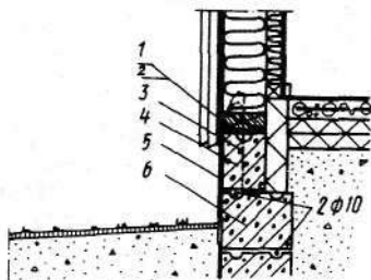
Рис. 99. Крепление наружной стеновой панели к бетонному фундаменту 1 — монтажный шов; 2 — слой гидроизоляции; 3 — закладной элемент для крепления каркаса; 4 — цокольный блок; 5 — отделочное покрытие цоколя; 6 — фундаментный блок
